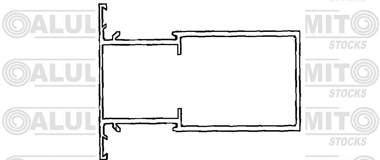
Pilastra Refuerzo Interior de 40*100
