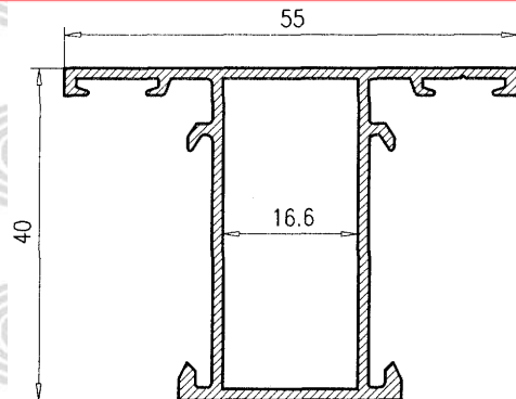
Pilastra 40*20
