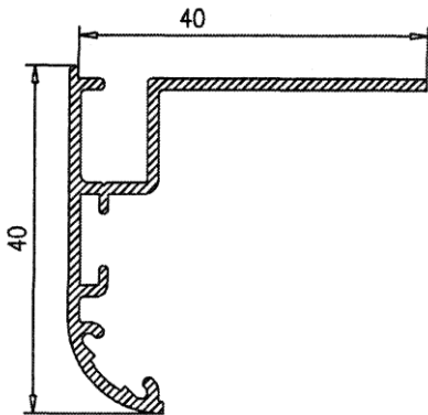
Premarco 40*40 031
