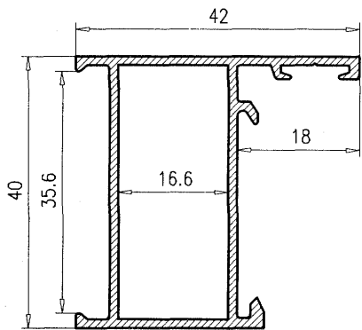
Marco 40*20
