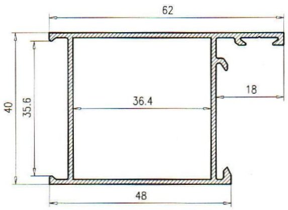
Marco 40*40 048
