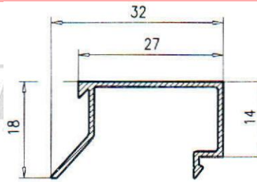
Junquillo Normal
