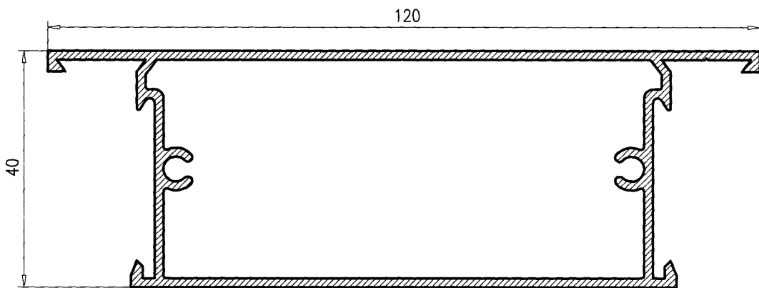
Pilastra Zócalo 120 415
