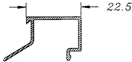
Junquillo 14
