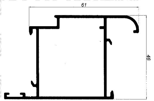
Hoja canto redondo 14
