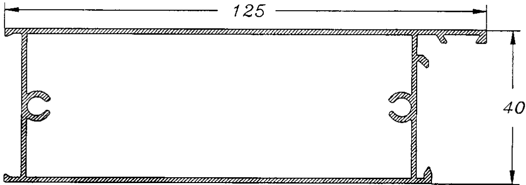
Marco Zócalo 362
