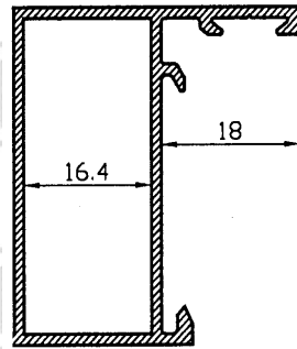
Marco celosía
