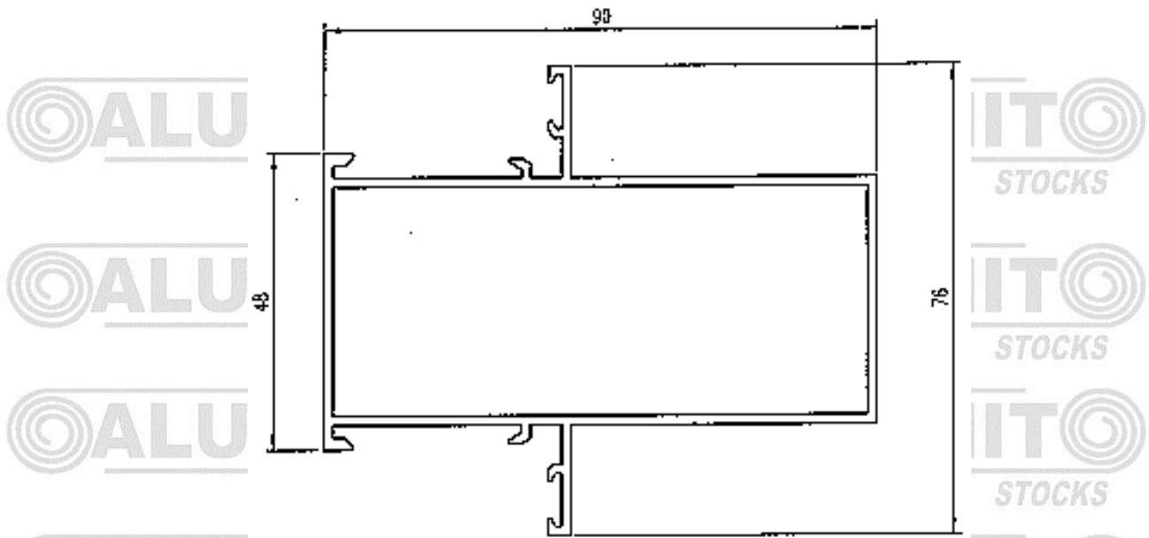
Pilastra Refuerzo Exterior de 40*90
