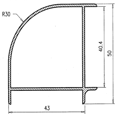
Esquinero 40
