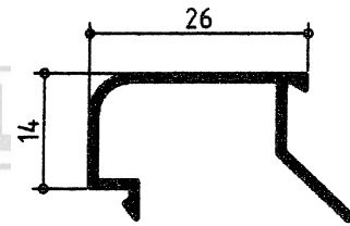
Junq. Normal Curvo
