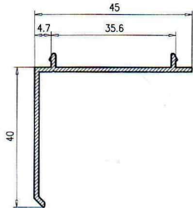
Premarco 40 040
