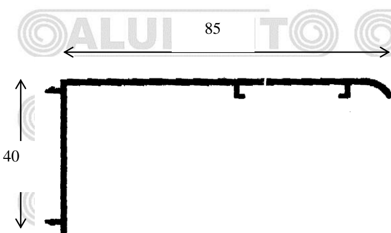
Premarco 85 061
