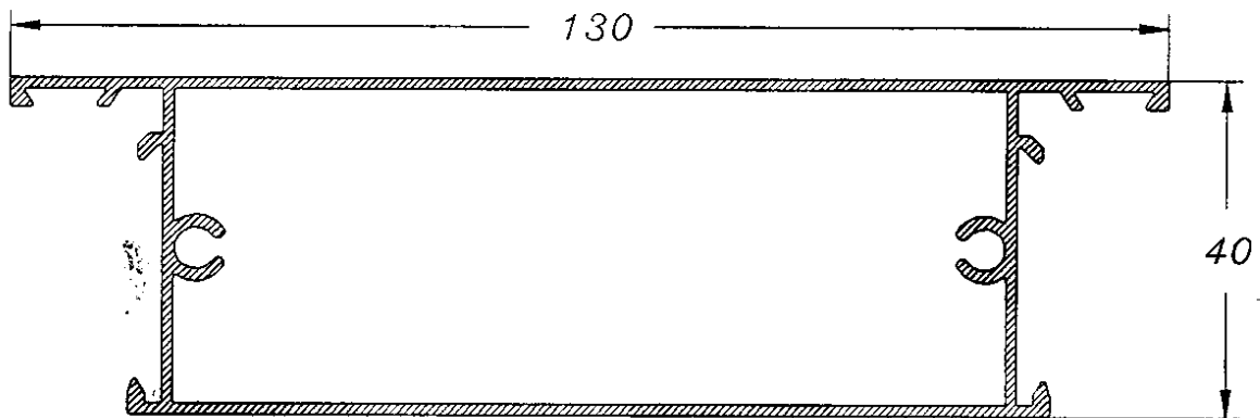
Pilastra Zócalo 416
