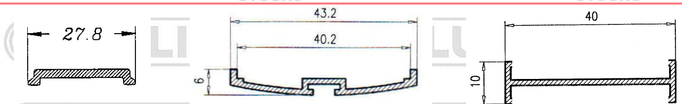
Pletina falleba
