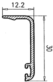
Premarco 40*40 031
