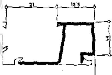
Junquillo Climalit
