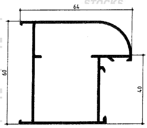
Marco Escaparate 050
