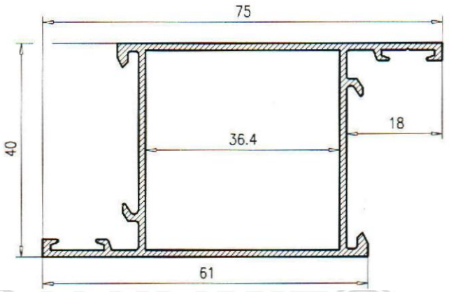
Hoja 40*40 944
