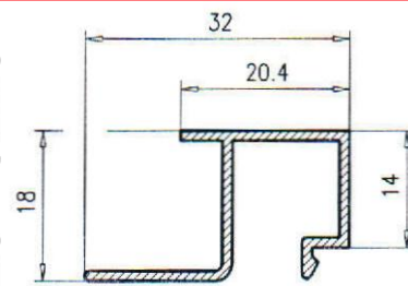
Junquillo 16
