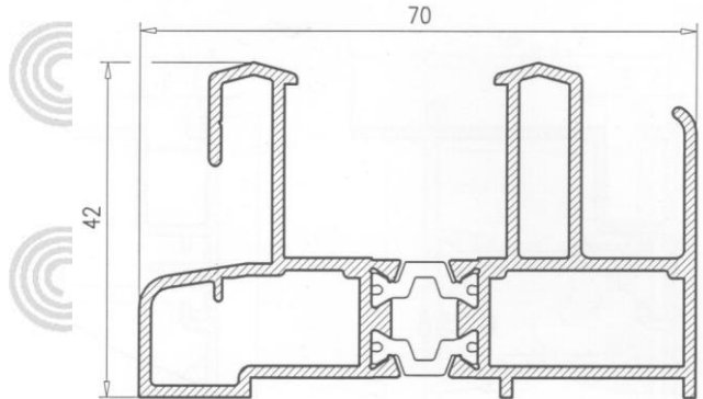
Marco de 70 Perimetral RPT 17200
