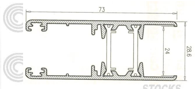
Hoja Multipunto Curva RPT
