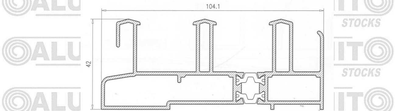
Marco 3 carriles RPT 17201
