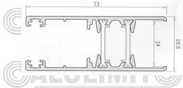
Hoja Climalit Multipunto RPT
