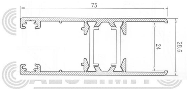
Hoja Climalit RPT
