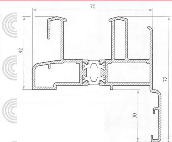
Marco de 70 Perimetral RPT 17200
