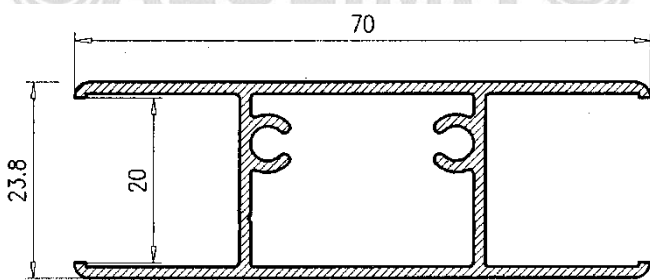
Parteluz Climalit
