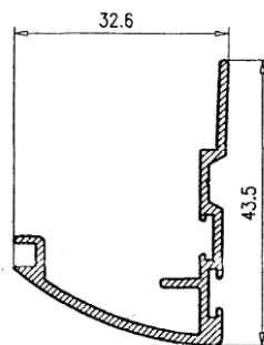
Suplemento 3 carriles 1820
