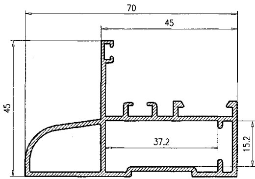
Marco Fijo 18818
