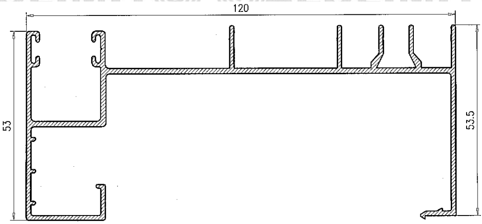
Marco Lateral con Guía de 120 derecha 706
