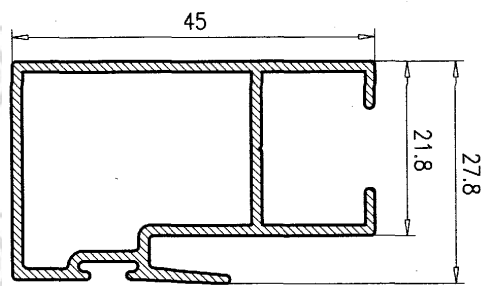
Hoja Central 45 7024
