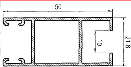
Hoja Lateral 50
