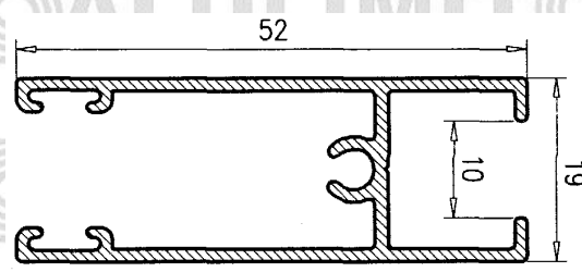
Hoja Rueda c/16 7018
