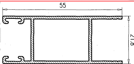
Hoja Lateral Climalit 55
