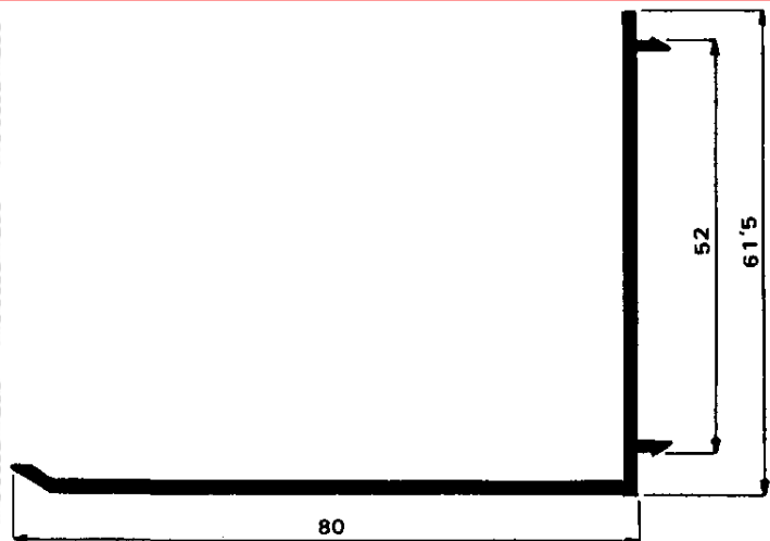
Premarco 80 060
