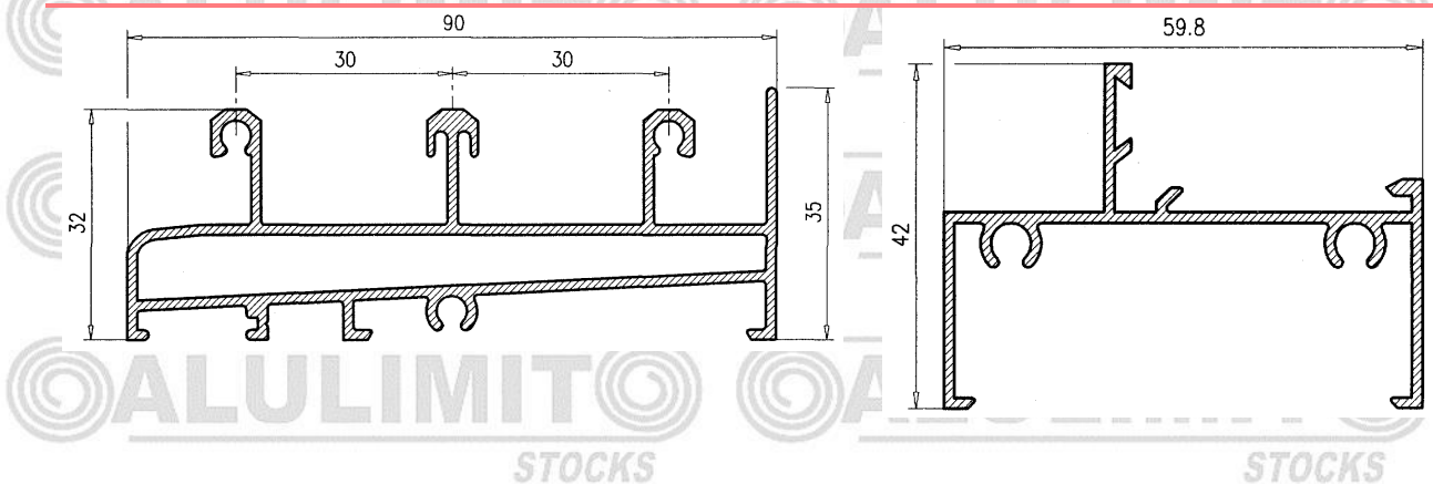
Marco Inferior 3 carriles
