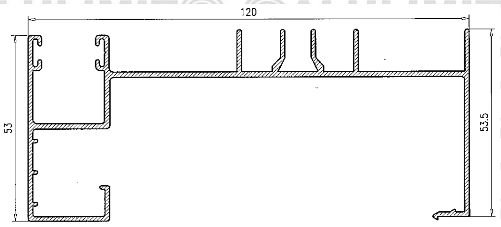
Marco Lateral con Guía de 120 izquierda 709
