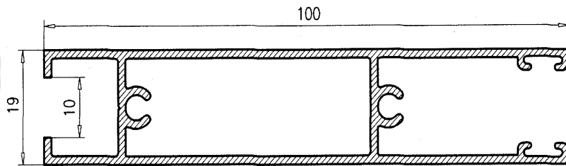
Zócalo Normal 7022
