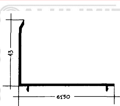
Premarco 30 042
