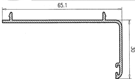
Premarco 30 042
