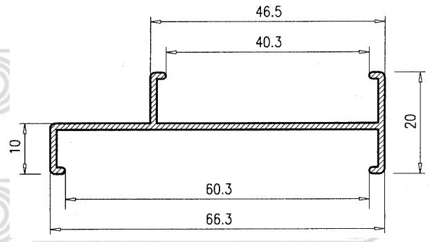
Union de 60 a 40 214
