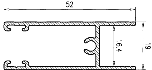
Hoja Central 50 7023
