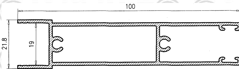
Zócalo Normal 7022
