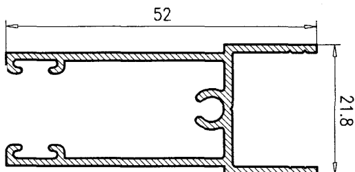
Hoja Central 50 c/16 7017
