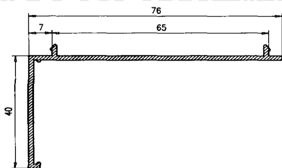
Premarco 40 045
