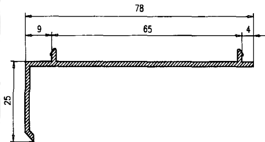
Unión Corredera 215
