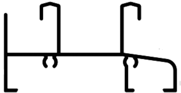
Marco Inferior sin cámara 124231
