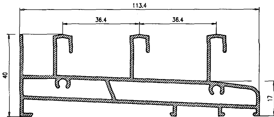
Marco Inferior 3 carriles
