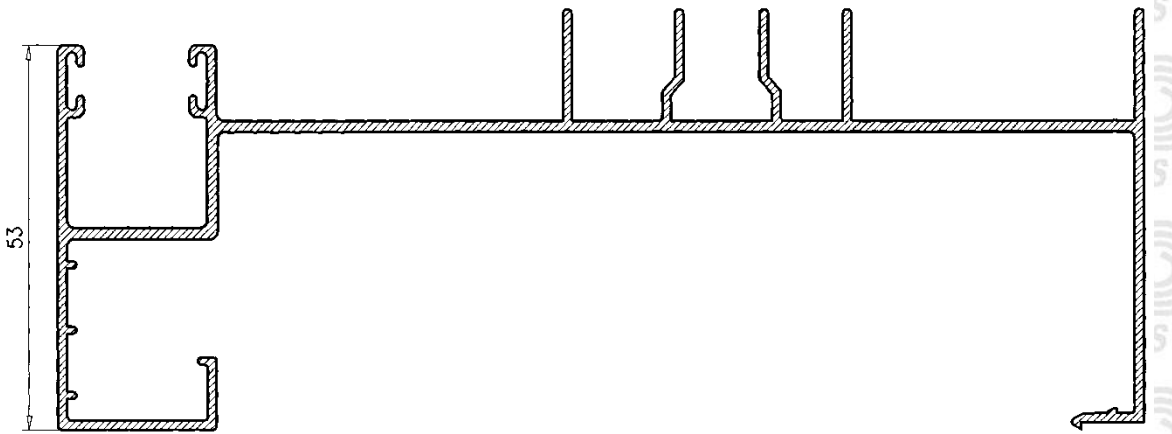
Marco Lateral con guía integrado Izquierdo 150
