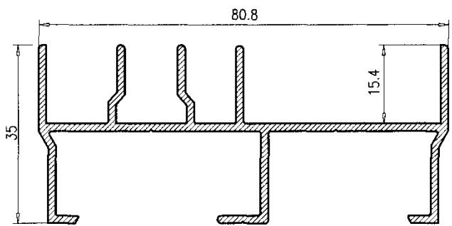
Marco Superior 124220
