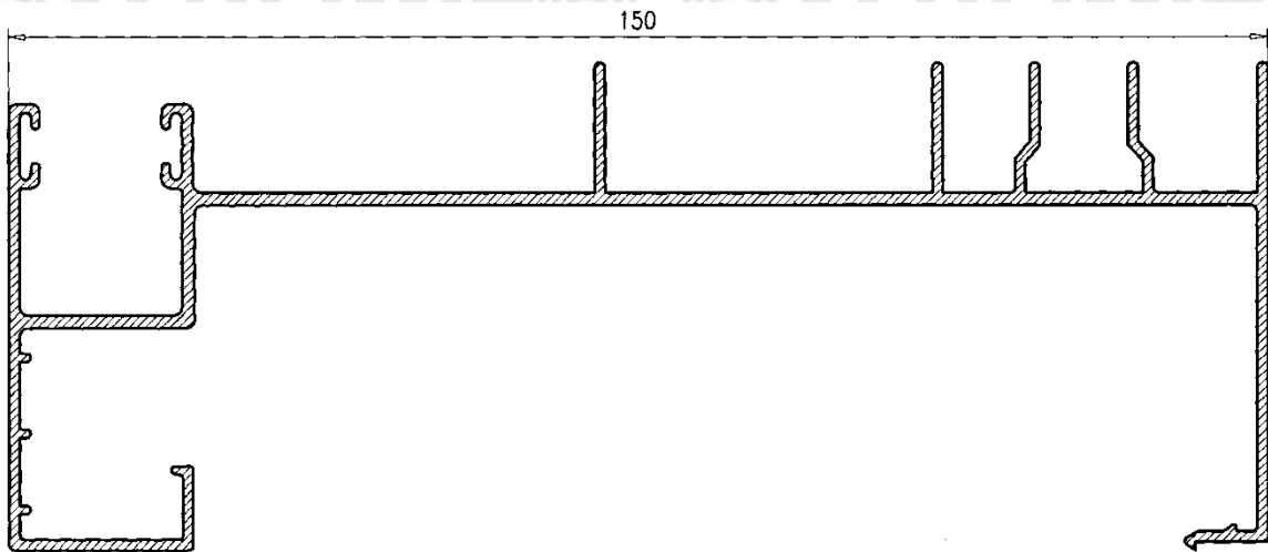
Marco Lateral con guía integrado Derecho 150
