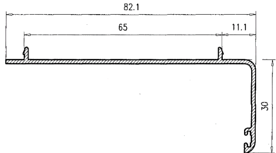
Premarco 30 036
