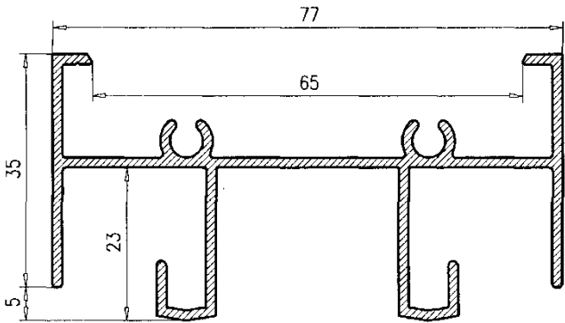
Marco Superior 124220
