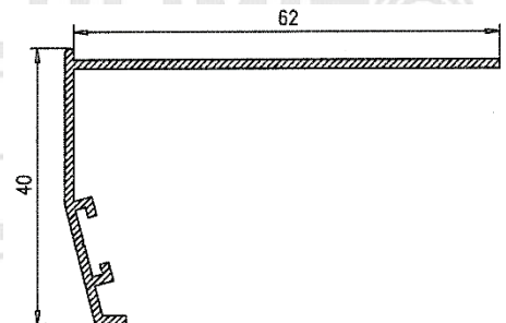
Solape 40 Recto 033
