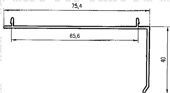
Premarco 40 biselado 046
