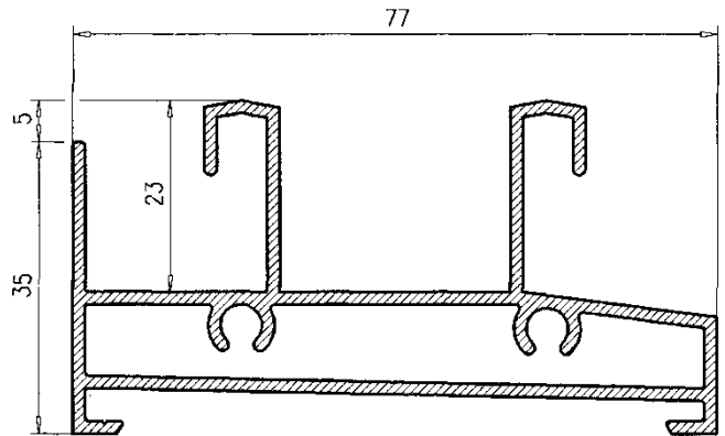
Marco Inferior 124230
