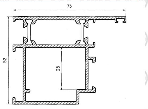
Marco Puerta Enrasado 26281
