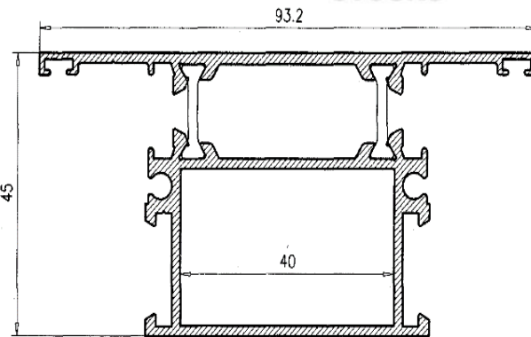
Pilastra Puerta 26580
