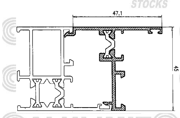
Marco Puerta Enrasado 26281
