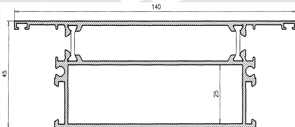
Pilastra Puerta 26580
