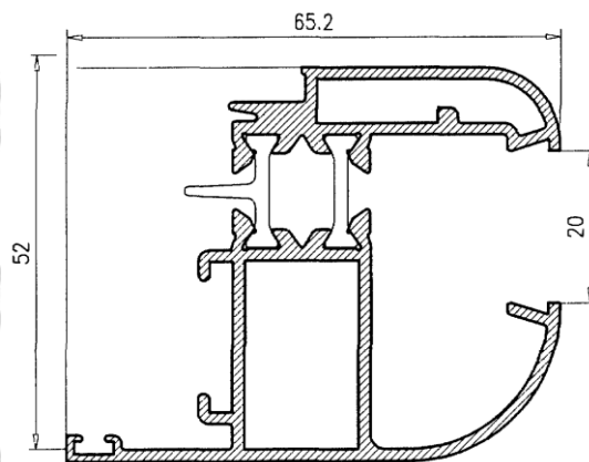
Hoja Ventana s/junq 25382
