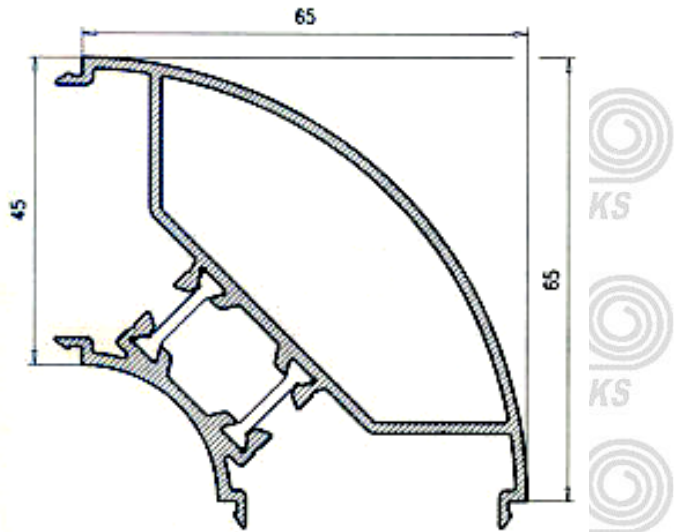
Esquinero 45 25092
