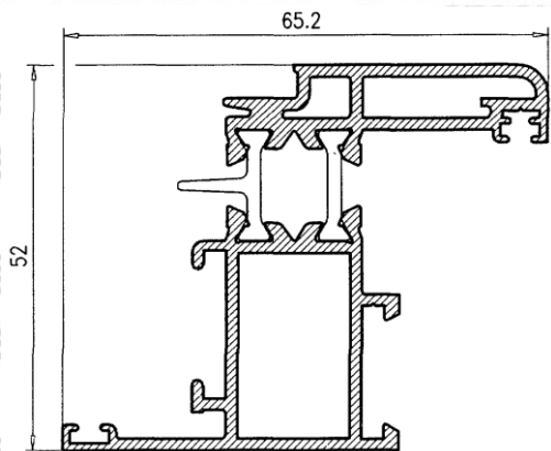
Hoja Enrasada Ventana 25380
