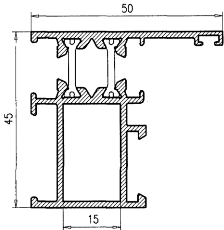
Marco Ventana 25280
