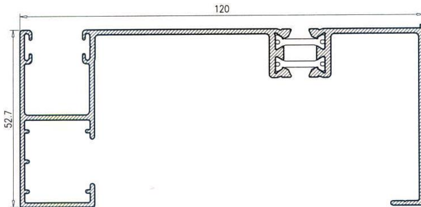
Pilastra Muro Cortina 26585
