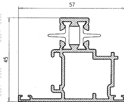
Perfil Pivotante 25284
