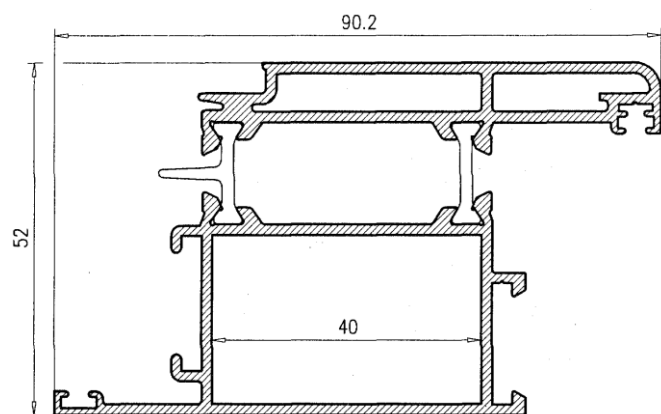
Marco Puerta 26280
