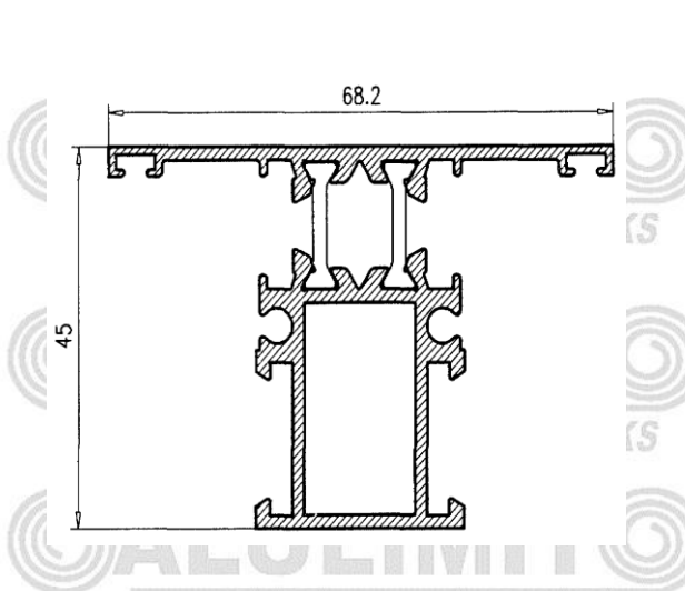
Pilastra Ventana 25583
