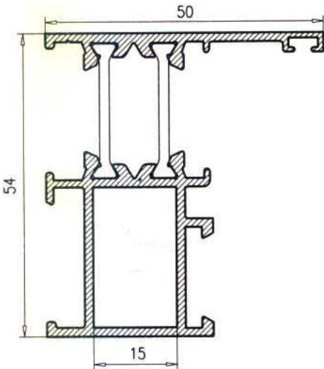
Marco Ventana 36280
