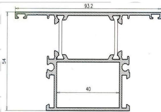
Pilastra Puerta
