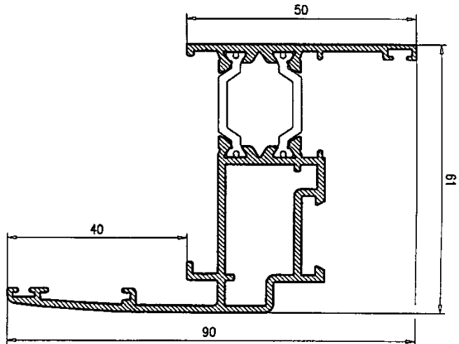
Marco Ventana con solape 36283
