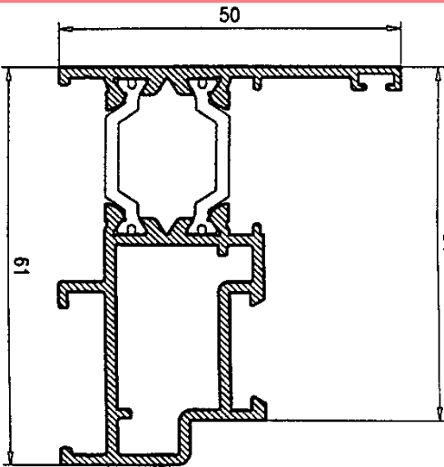
Marco Ventana 36279
