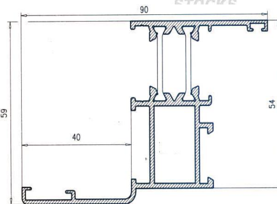
Marco Ventana Solape 36281
