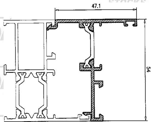
Inversor de marco 36384
