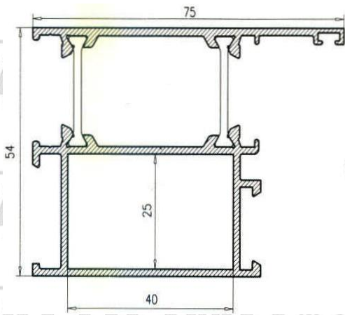
Marco Puerta
