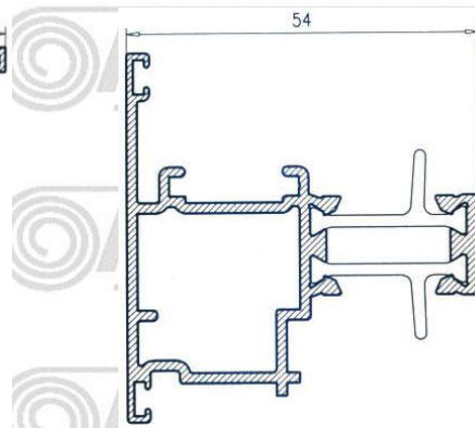
Pivotante
