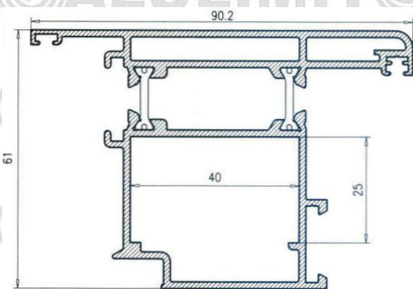
Hoja Apertura Exterior Puerta
