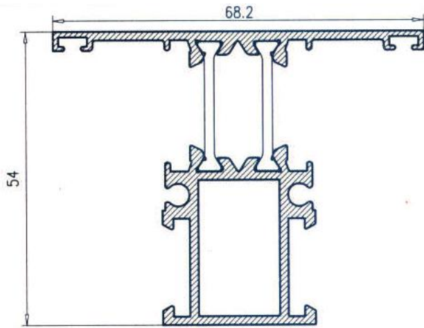
Pilastra Ventana 36580
