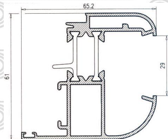
Hoja Ventana s/junquillo 36282
