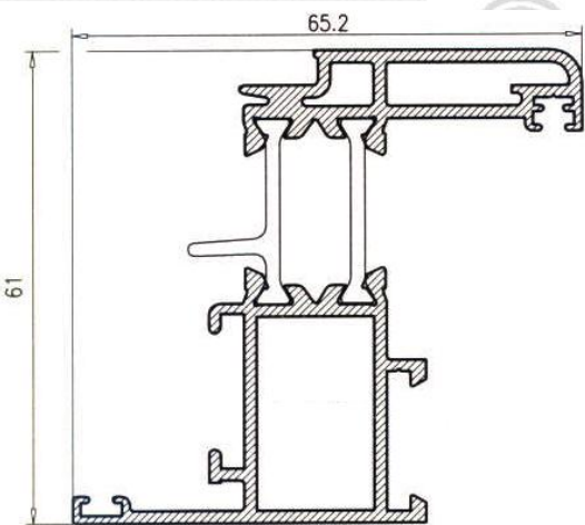
Marco Ventana 36380
