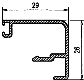
Junq. Base 29 hueco 21.5 36262
