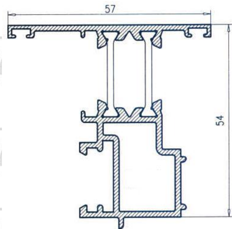
Esquinero 45 36381
