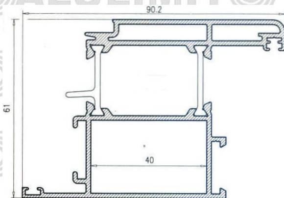
Hoja Puerta
