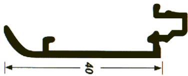
Premarco 40 7240
