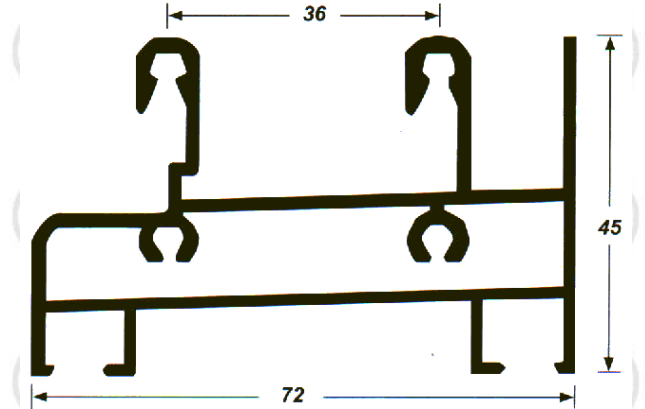
Marco Inferior 7201
