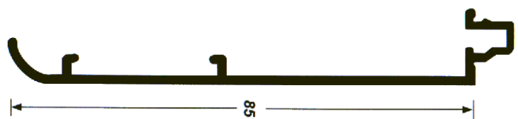
Premarco 85 7285
