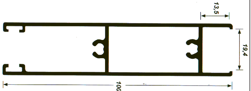
Zócalo Climalit 7220
