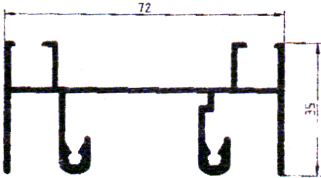
Marco Superior 7202
