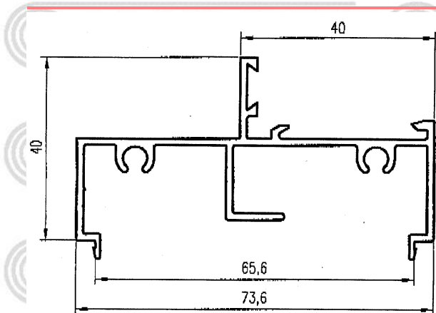
Marco Inferior c/refuerzo 812
