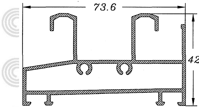
Marco Lateral c/pestaña 803
