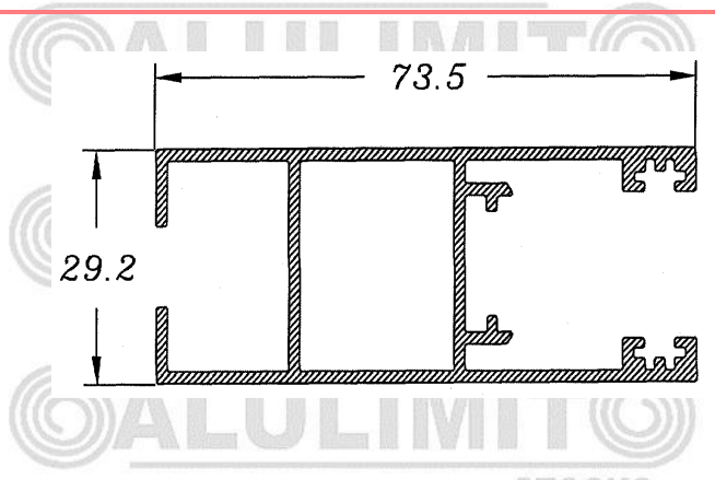
Marco Superior c/refuerzo 811
