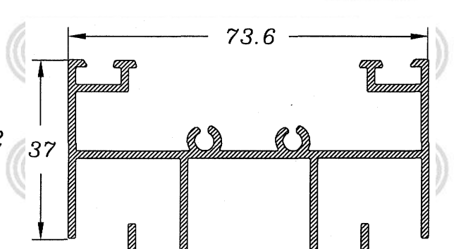
Marco Lateral c/refuerzo 813
