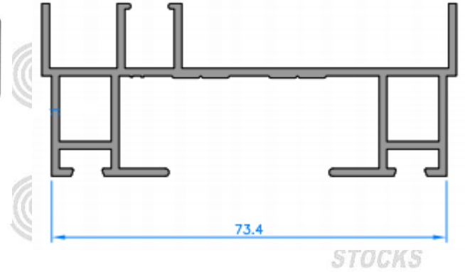
Marco Lateral c/refuerzo 813
