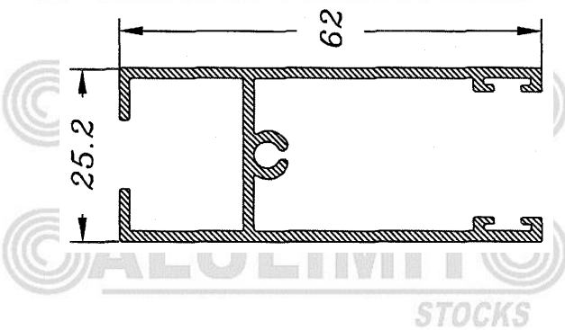
Hoja Rueda Normal 806
