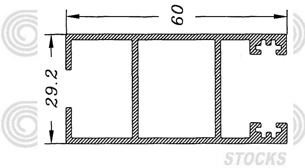
Hoja Lateral Normal 804
