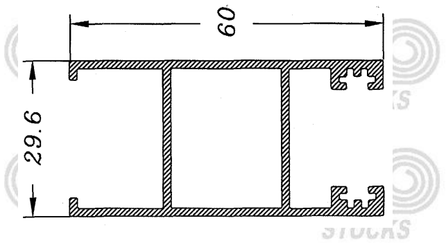
Hoja Lateral Climalit 834
