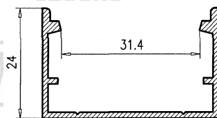
Forma U 25
