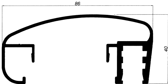
Pasamano 86 europeo acristalar 320 STOCKS
