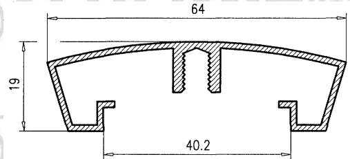
Pasamano autorroscado
