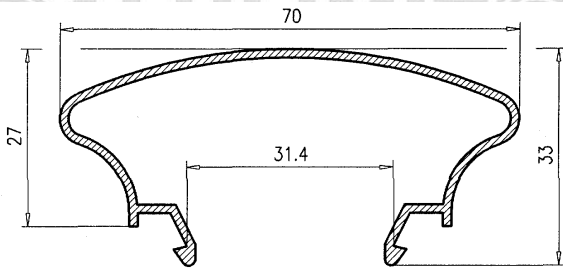
Pasamano Barandilla
