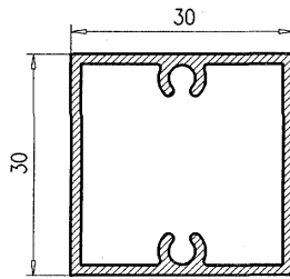
Cuadrado 30 aut.
