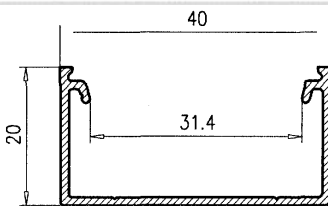
Forma U 20
