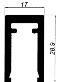
U para acristalar 810 STOCKS
