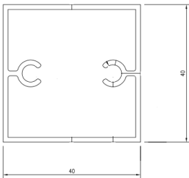
Cuadrado 40 aut.
