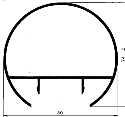
Pasamano Redondo 80
