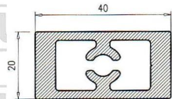
R. 40*20 aut.
