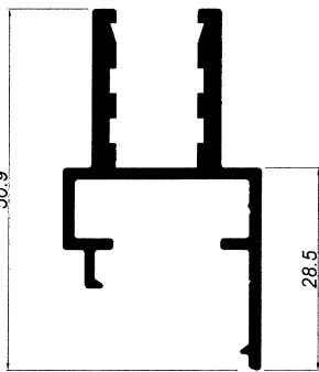
Anclaje Cristal 797 STOCKS
