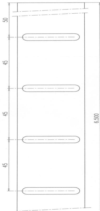
Montante paso 45 mm 22 LAMAS / METRO
