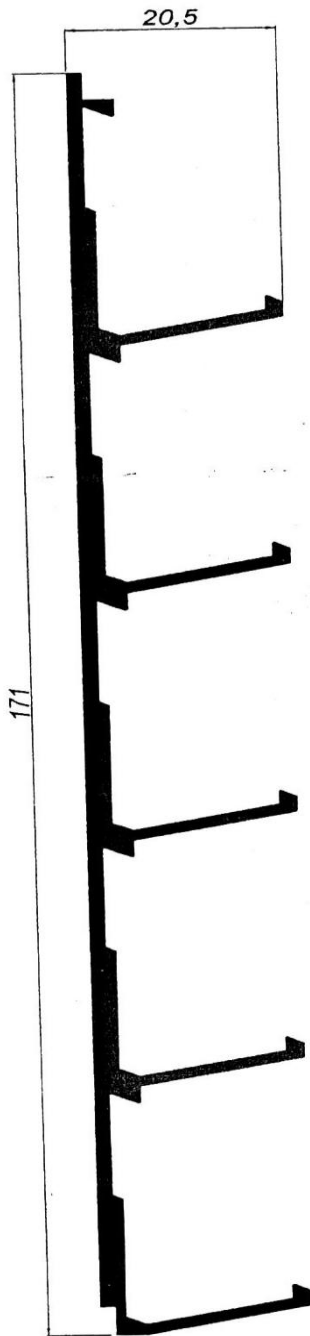
Soporte Lama Peine 171 915
