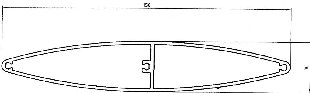
Lama ala Avión 150 2856
