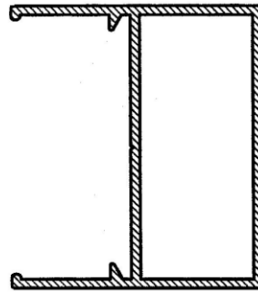
Montante 100 troquelado paso 0 24T
