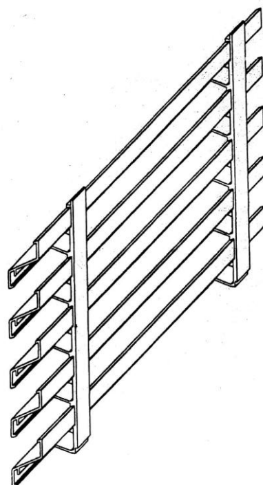
Esquema de montaje de la LAMA y el SOPORTE
