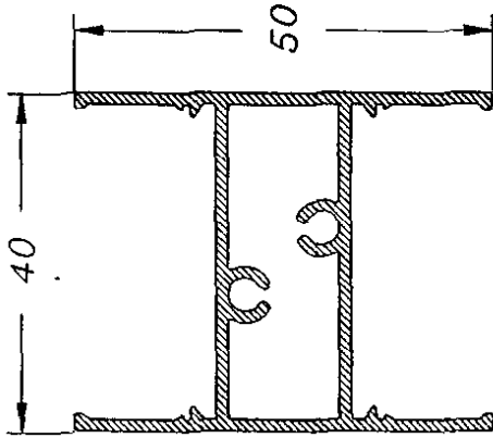
Parteluces
