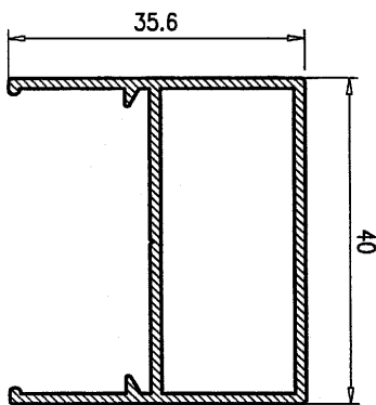
Marco Celosía 24
