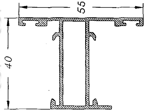
T inversora
