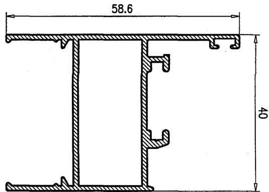
Hoja europeo 25
