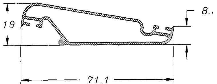
Lama Perla 70
