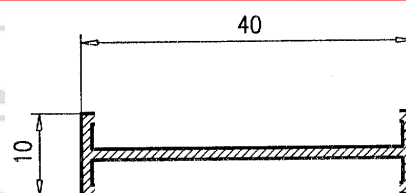
Unión 40
