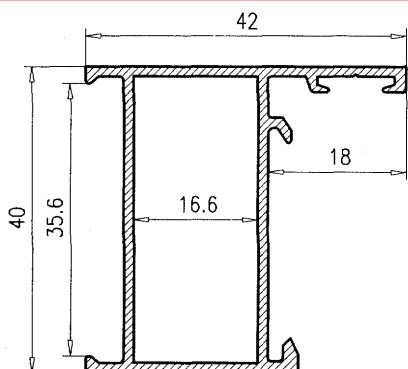
Marco 40*20
