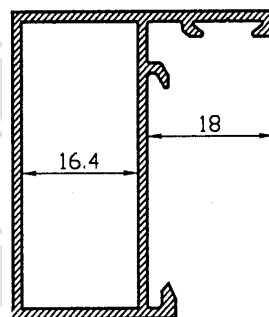
Marco celosía
