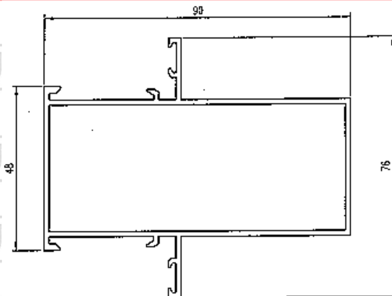
Pilastra Refuerzo Exterior de 40*90
