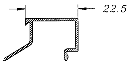
Junquillo 14
