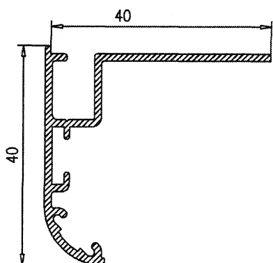
Premarco 40*40
