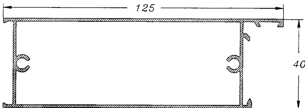
Marco Zócalo
