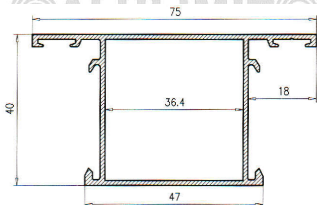
Pilastra 40*40
