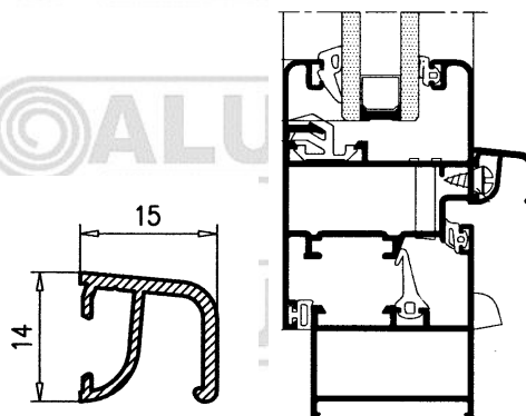
Vierteaguas hoja Recojecondensaciones
