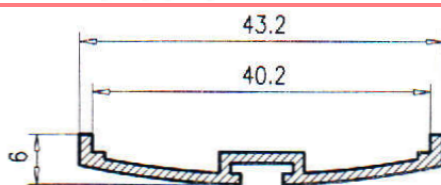
Perfil Vaivén
