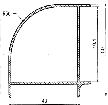
Esquinero 40
