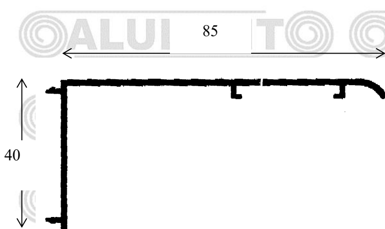
Premarco 85
