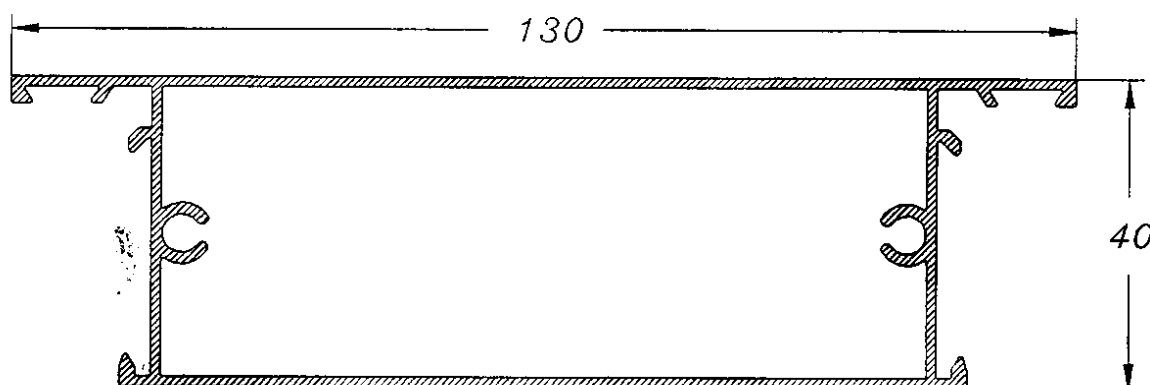
Pilastra Zócalo
