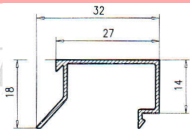
Junquillo Normal
