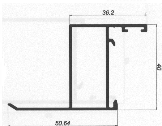
Marco con solape biselado
