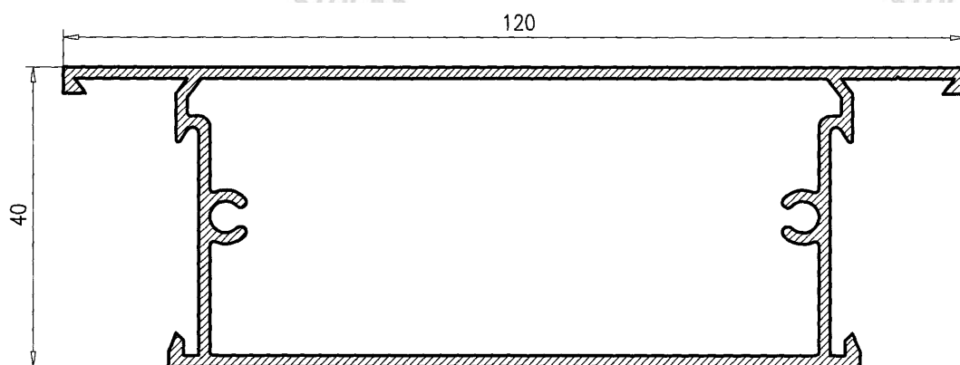
Pilastra Zócalo 120
