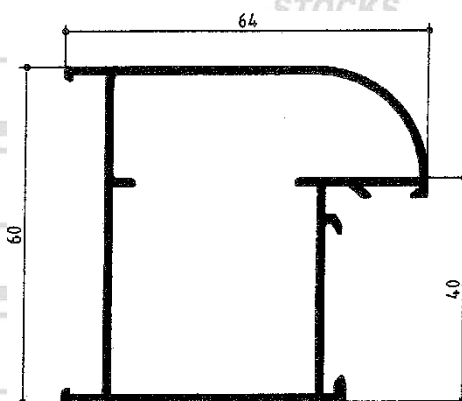
Marco Escaparete
