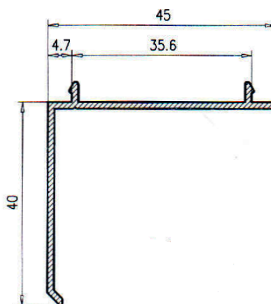
Premarco 40
