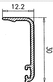
Premarco Cajón 30
