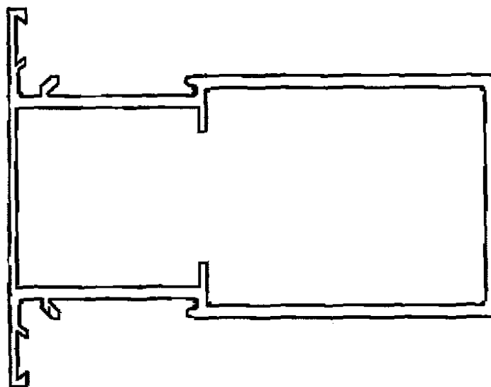
Pilastra Refuerzo Interior de 40*100
