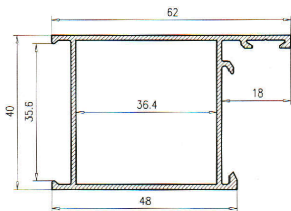
Marco 40*40
