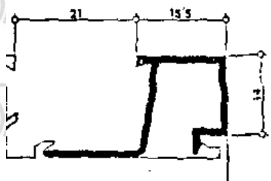
Junquillo Climalit
