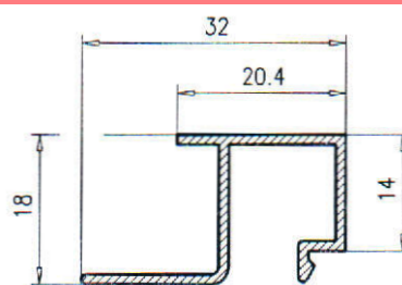
Junquillo 16
