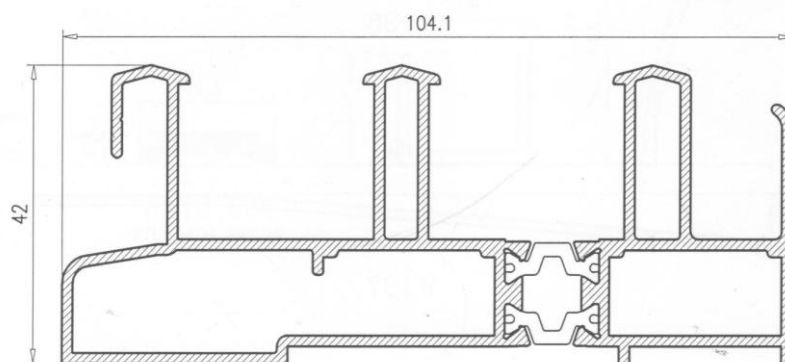
Marco 3 carriles RPT 17201
