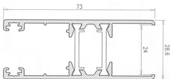
Hoja Climalit RPT
