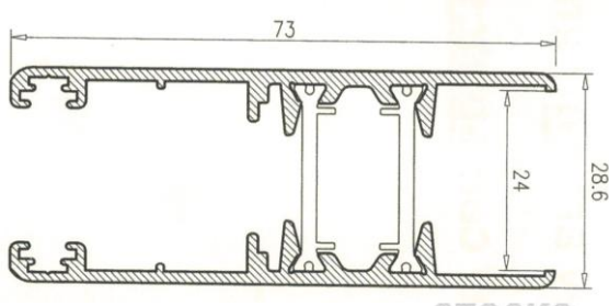
Hoja Multipunto Curva RPT
