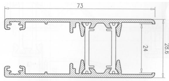
Hoja Climalit Multipunto RPT
