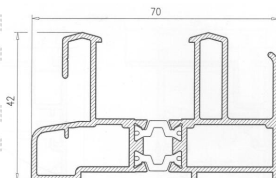
Marco de 70 Perimetral RPT 17200
