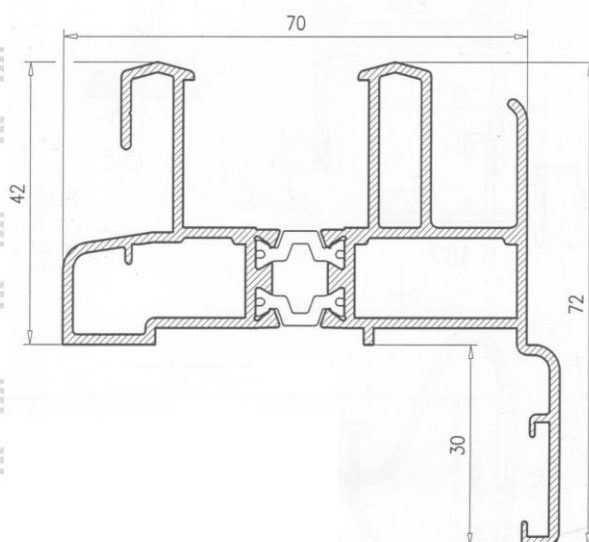
Marco de 70 Perimetral RPT 17200
