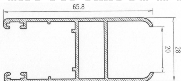
Hoja Curva Climalit
