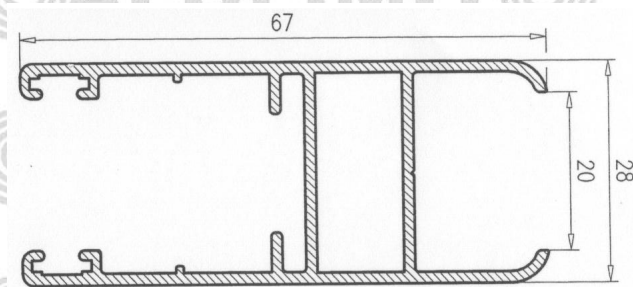
Hoja Multipunto c-20
