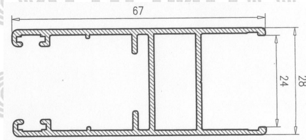
Hoja Multipunto c-24
