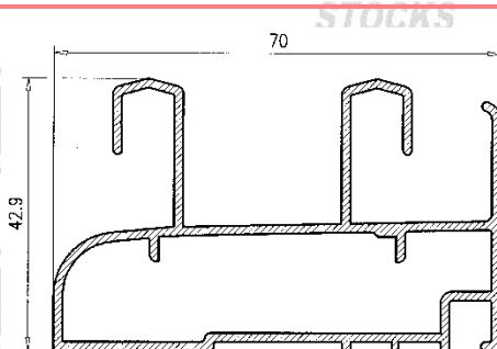
Marco de 70 Perimetral
