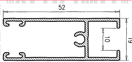
Hoja Rueda
