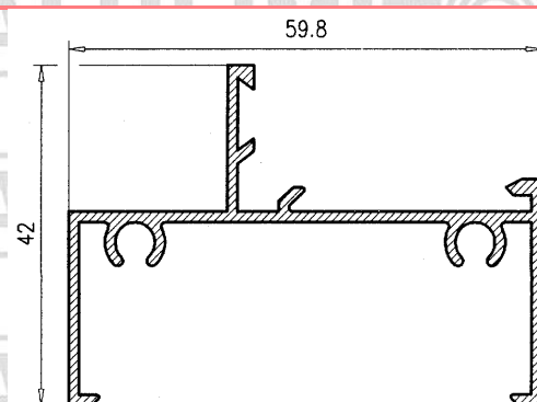
M. Fijo Hembra
