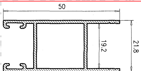
H. Lateral Climalit 50
