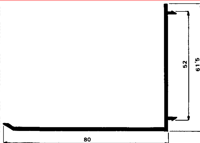
Premarco 80 060
