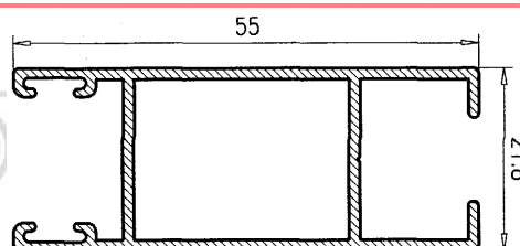
Hoja Lateral 55
