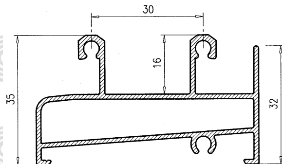
Marco Inferior
