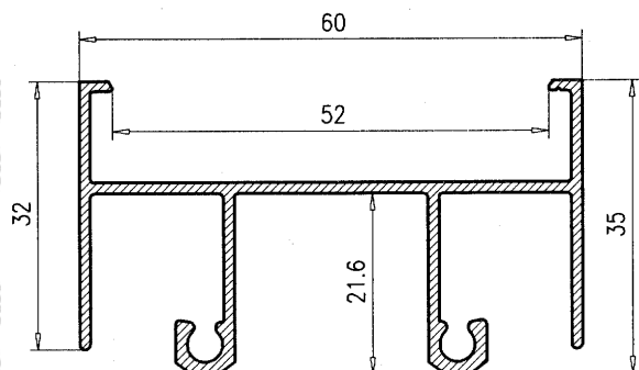
Marco Superior
