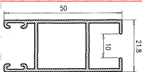
Hoja Lateral 50
