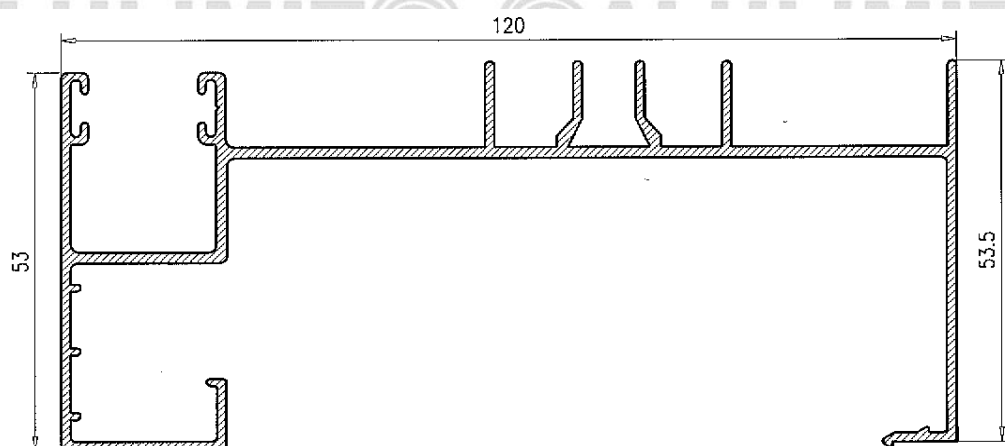
Marco Lateral con Guía de 120 izquierda
