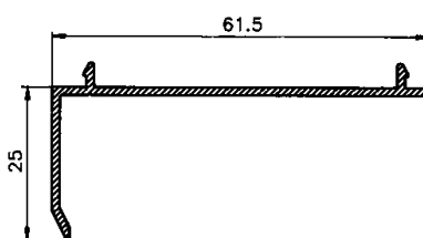
Premarco 50 044
