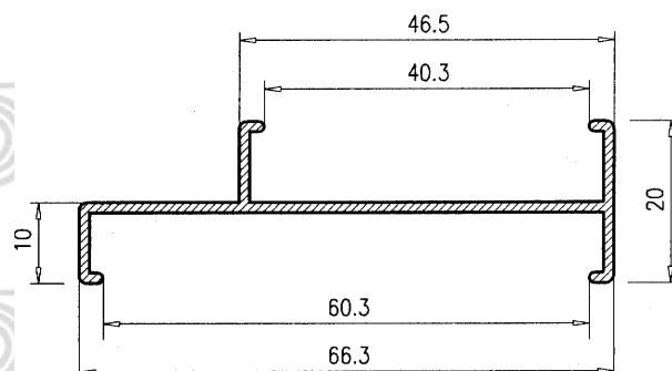
Union de 60 a 40
