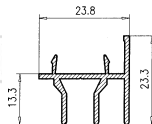
Hoja Cierre 4 hojas 19
