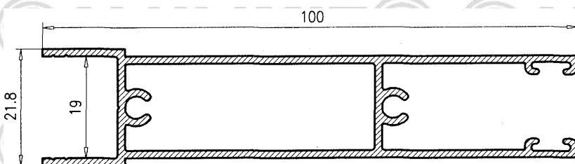
Zócalo Normal 7022
