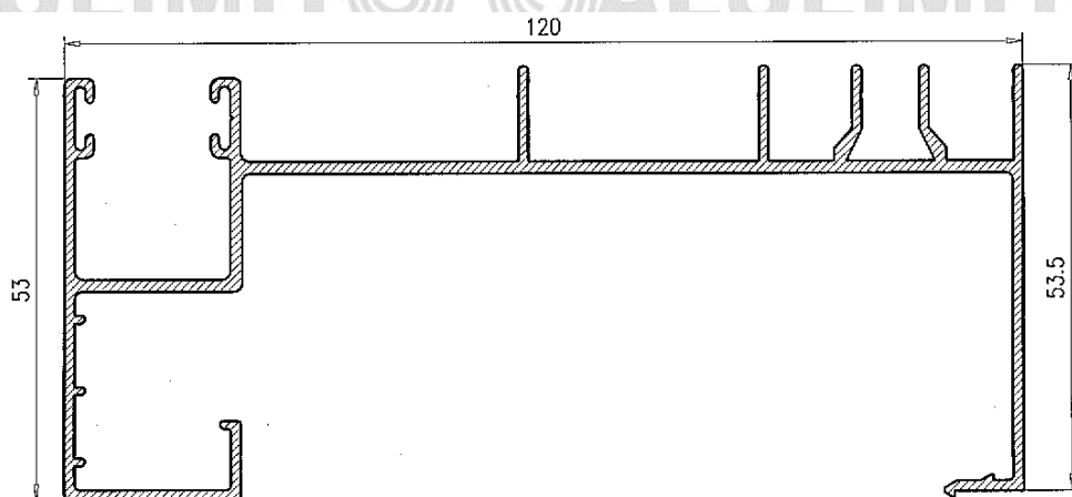
Marco Lateral con Guía de 120 derecha
