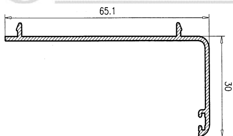
Premarco 30 042
