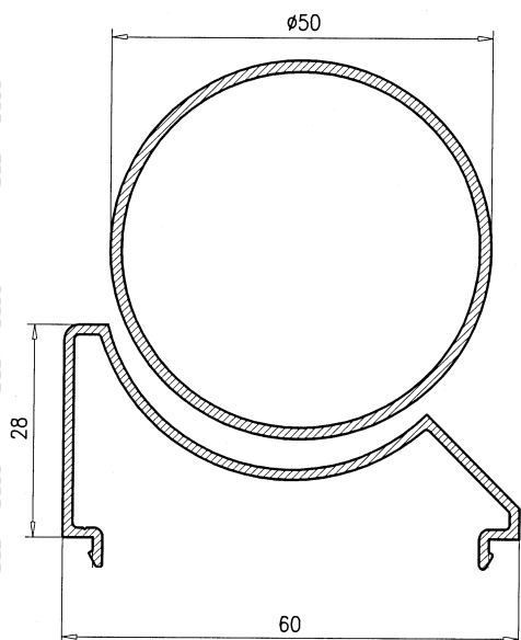
Rotula 60 7000
