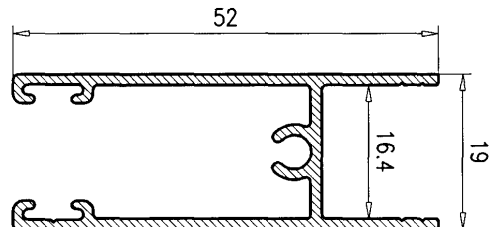
Hoja Rueda c/16
