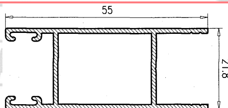
Hoja Lateral Climalit 55
