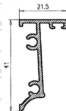
Marco Inferior 123486
