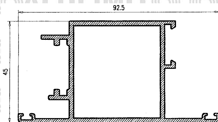
Hoja Apertura Exterior 123482
