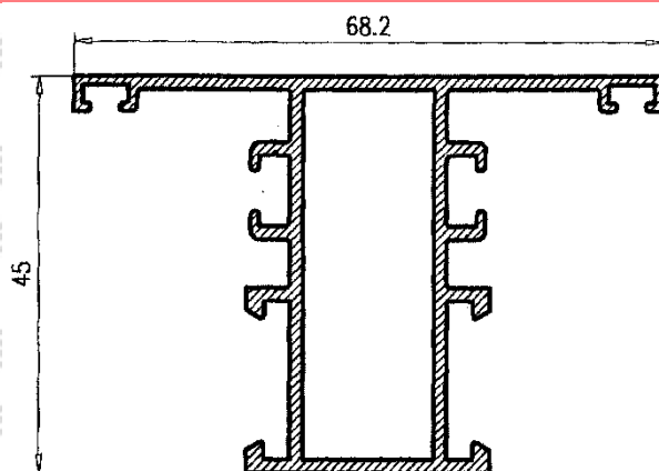
Hoja Ventana s/junquillo c/20 122383
