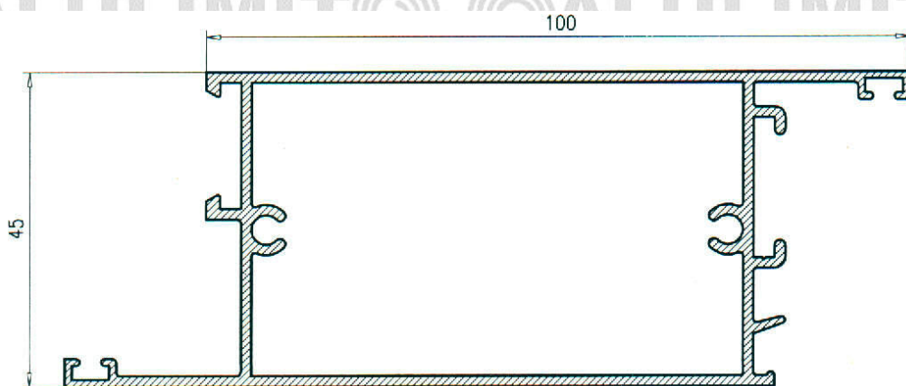
Hoja Zócalo 123477
