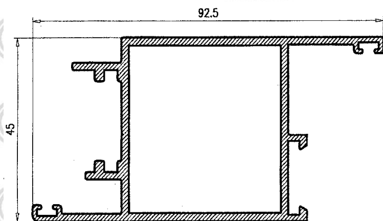
Hoja Apertura Interior 123481
