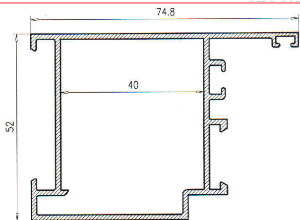
Marco Puerta C40/ Enrasado 123282
