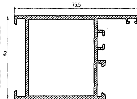
Marco Puerta Cámara 40 123281
