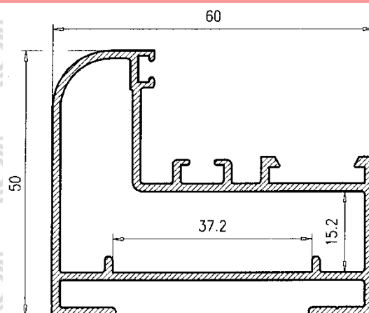
Marco Escaparate 121283
