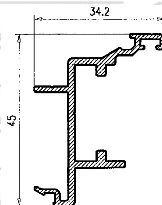
Marco apertura Interior para Fijo 123484
