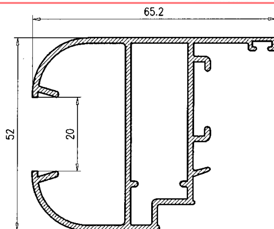
Hoja Ventana s/junquillo c/20 122383
