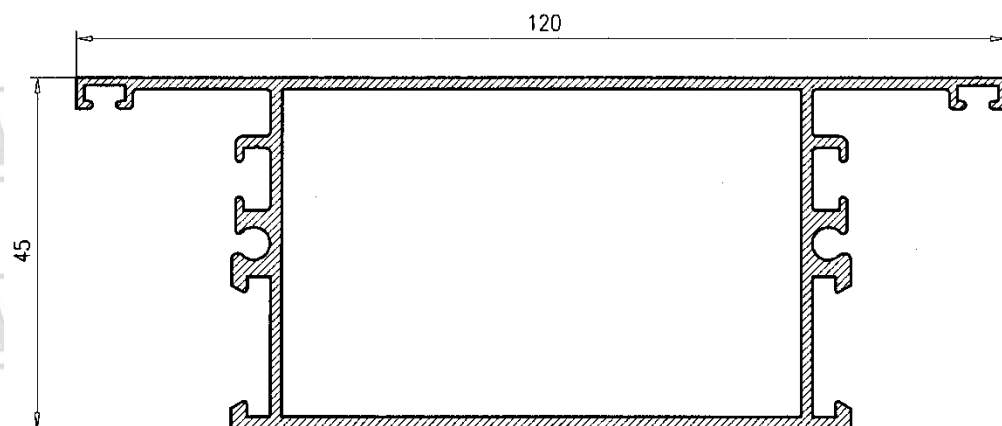
Pilastra Zócalo 123478
