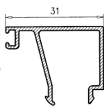
Junq. Base 31 de ja hueco 10 122716
