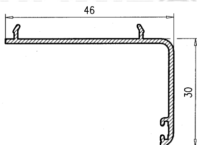
Premarco 30 041
