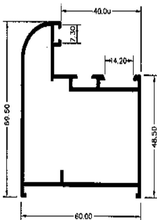
Marco Escaparte 74 123284
