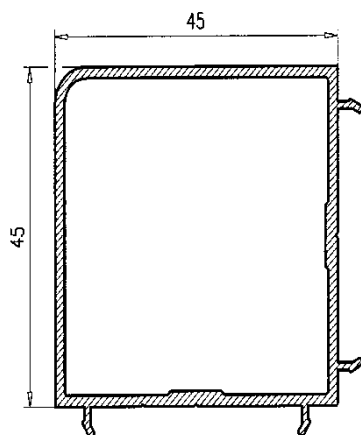
Esquinero 90 7058
