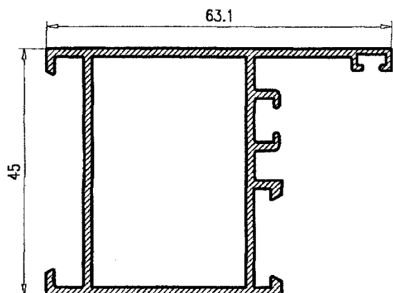
Marco Puerta 123280
