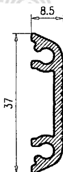
Marco Inferior Liso 123487
