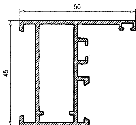
Marco Ventana 122280
