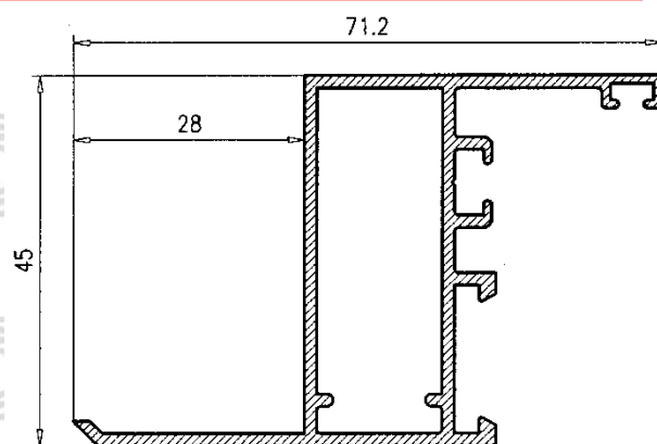
Marco con Solape 122281
