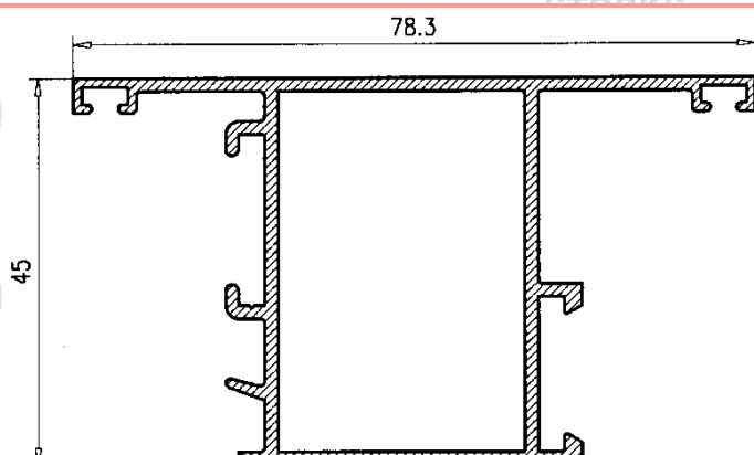
Hoja Puerta Apert. Ext. Clásica 123584
