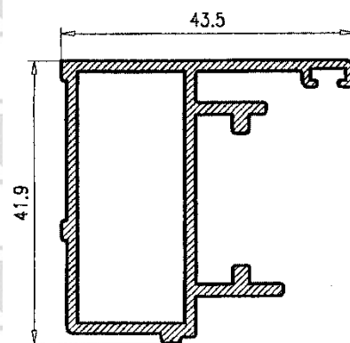
M. Apert. Exterior para Fijo 123485
