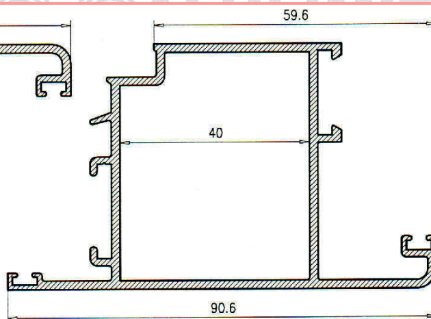
H. Puerta Aper. Ext C/40 123583
