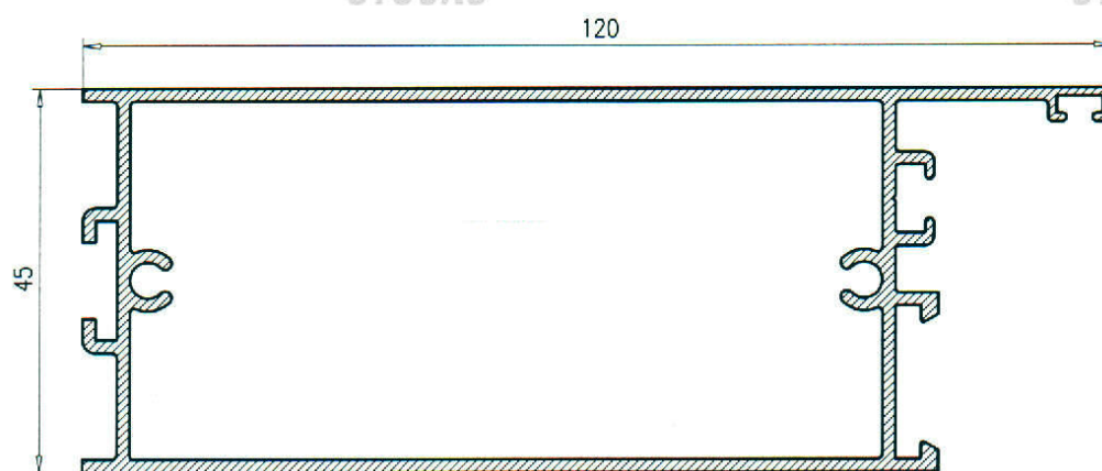
Marco Zócalo 123476
