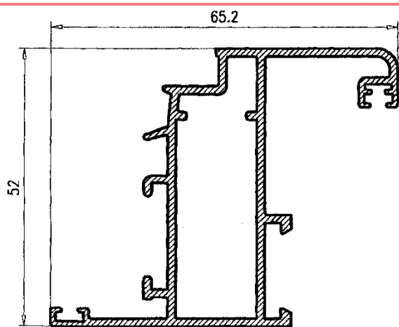
Hoja Enrasada Ventana 122382
