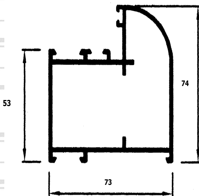
Marco Escaparte 73 121285
