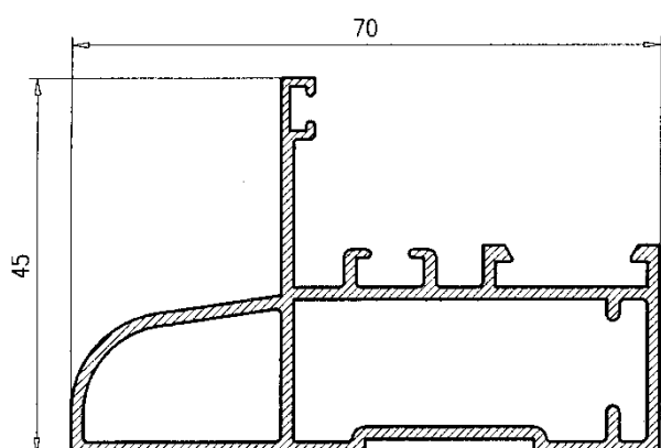
Perfil Pivotante 122084
