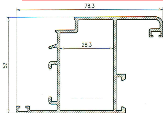
Hoja Enrasada Puerta 123381
