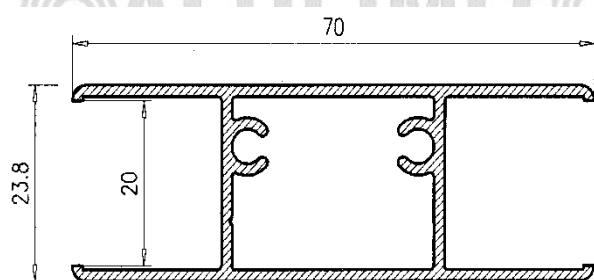
Parteluz Climalit 116217
