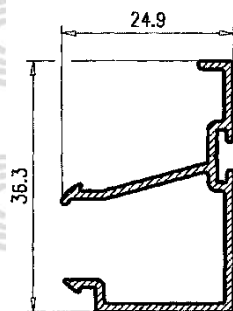
Junquillo Vaivén 122714
