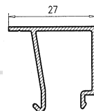
Junq. Base 27 de ja hueco 14 122715
