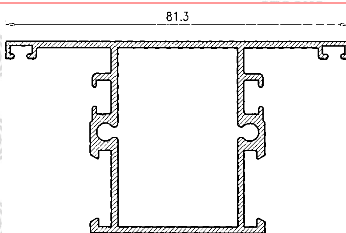
Pilastra Puerta Autorroscada 123581
