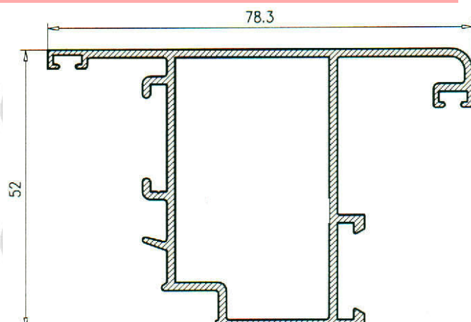
H. Puerta Apertura Exterior 123582
