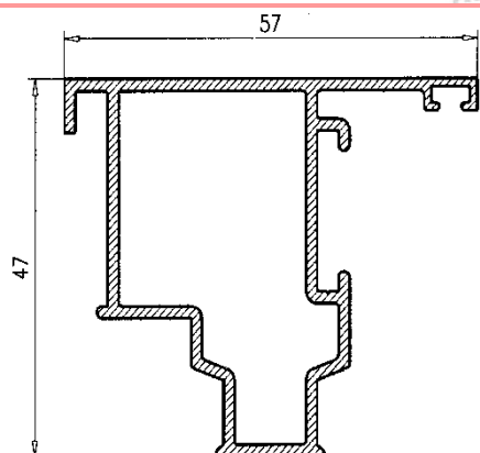
Perfil Pivotante 122084
