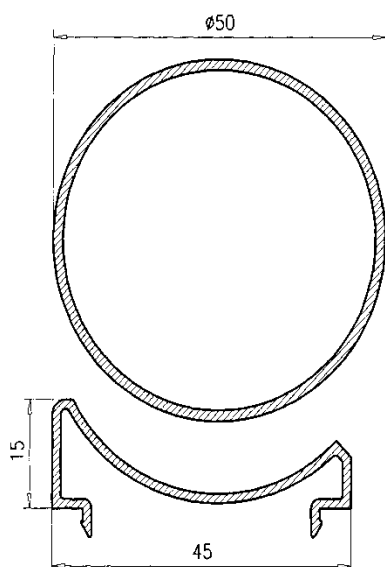
Rotula Abatible 45 122722
