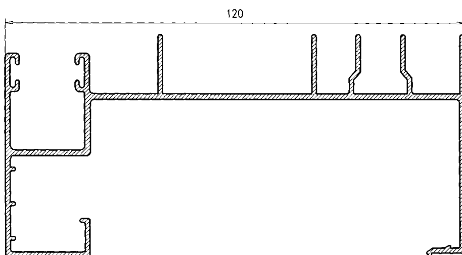
Marco Lateral con guía integrado Derecho 120
