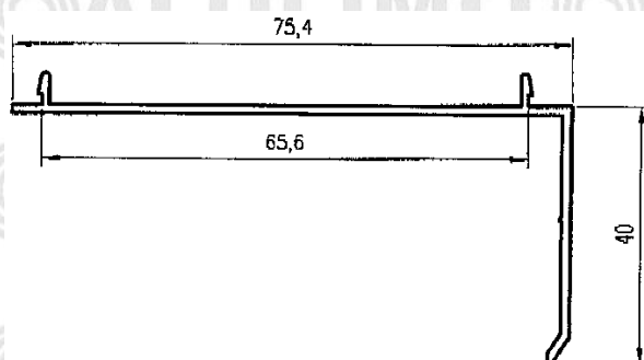
Premarco 40 biselado
