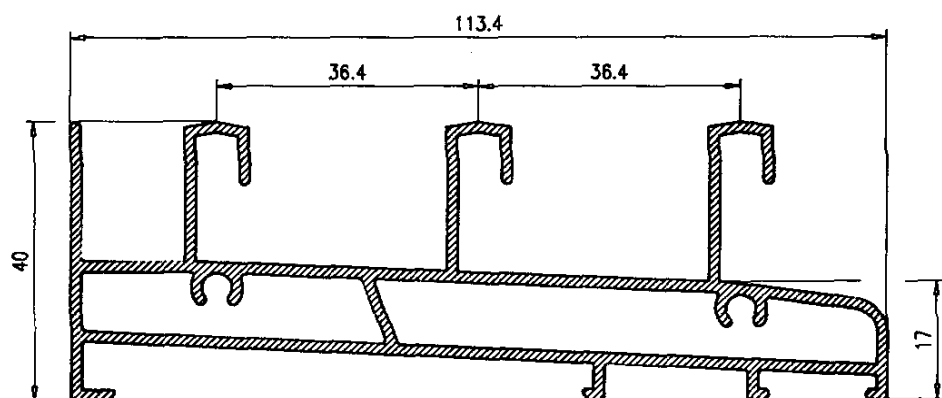
Marco Inferior 3 carriles
