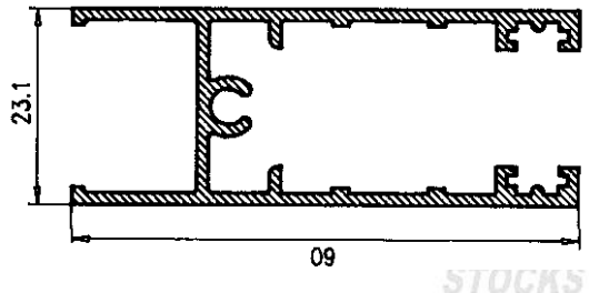
Hoja Rueda Climalit 124351
