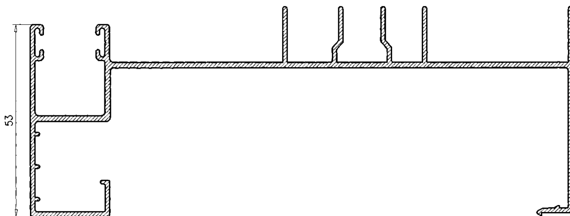
Marco Lateral con guía integrado Izquierdo 150 2450
