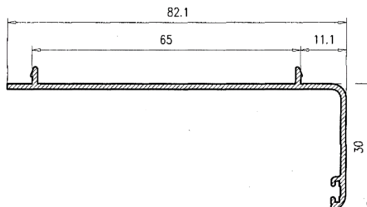
Premarco 30
