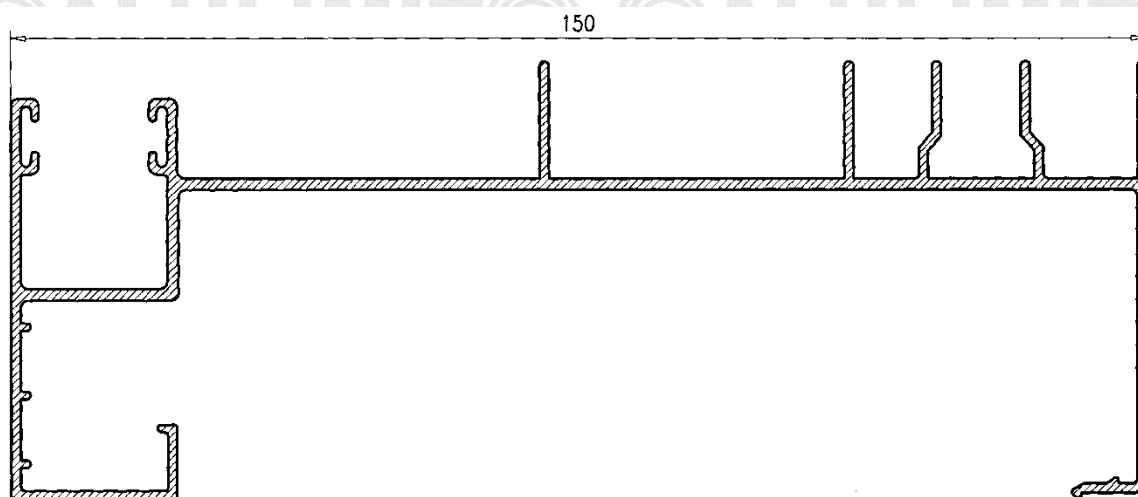
Marco Lateral con guía integrado Derecho 150 2451
