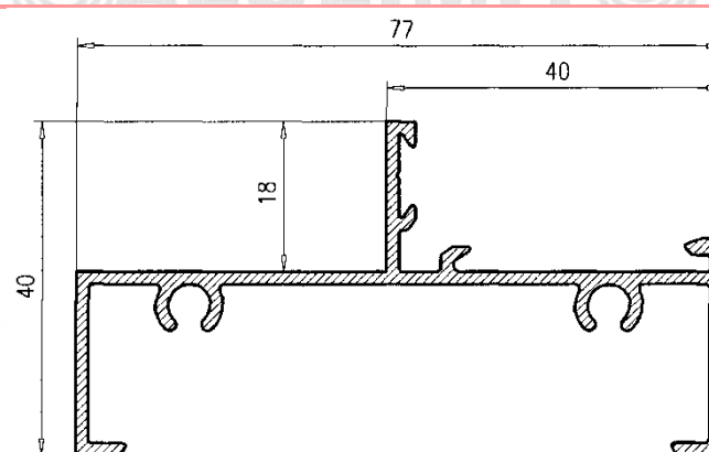
Marco Fijo Hembra 904
