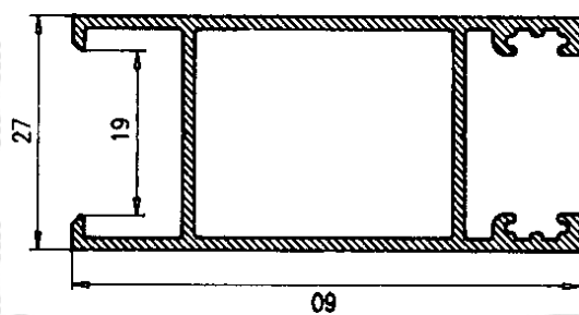
Hoja Lateral Climalit 124312
