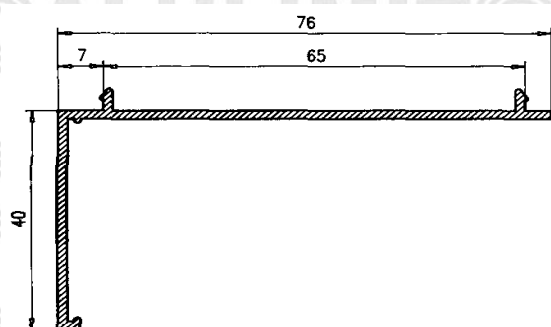
Premarco 40
