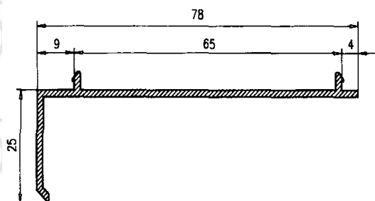
Premarco 25
