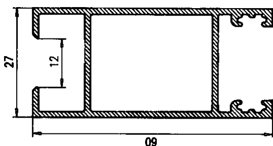
Hoja Lateral 124310
