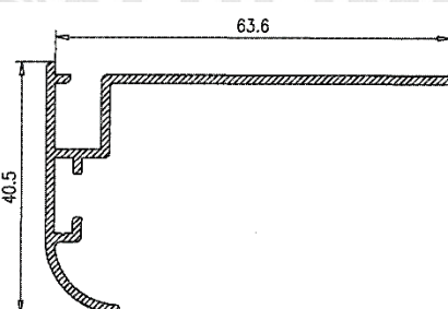
Solape 40 Cataluña
