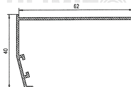
Solape 40 Recto
