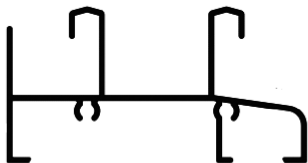
Marco Inferior sin cámara 124231
