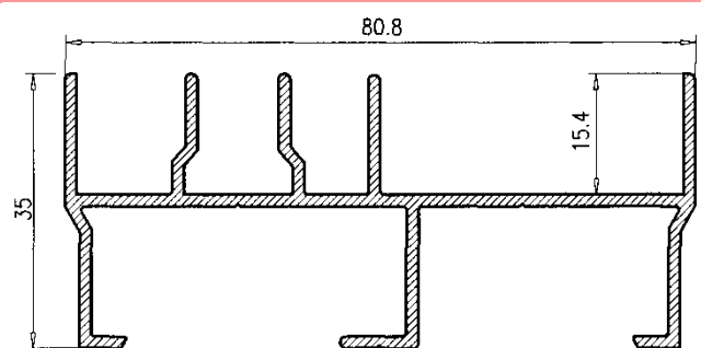
Marco Superior 124220
