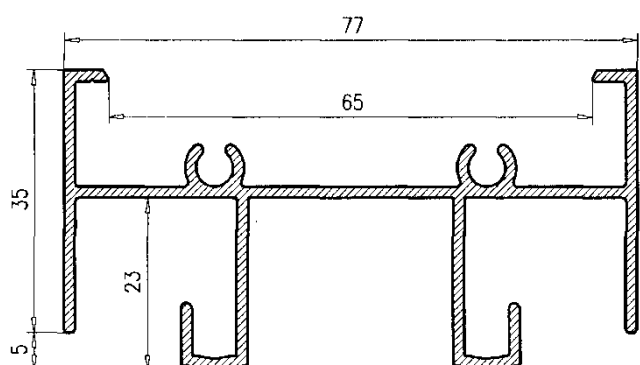
Marco Superior 124220
