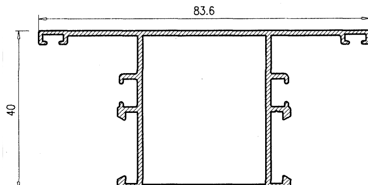
Pilastra Puerta 129580
