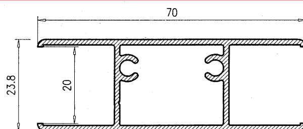
Parteluz Climait 116217
