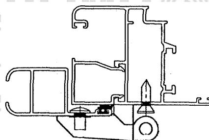
Contraventana 122080
