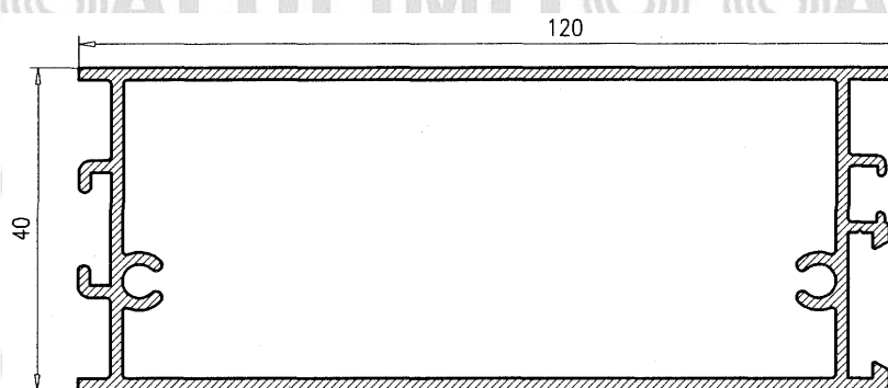
Marco Zócalo 129476
