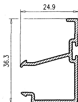
Premarco 40 040
