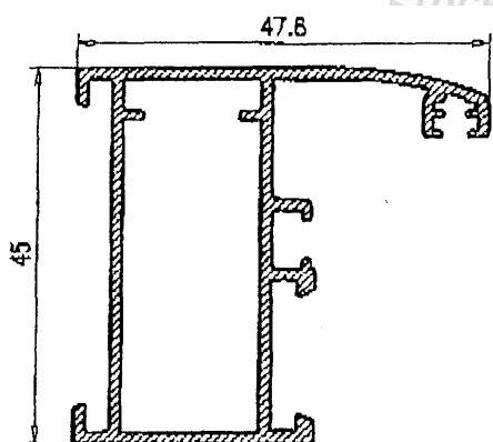
Hoja Enrasada 28380
