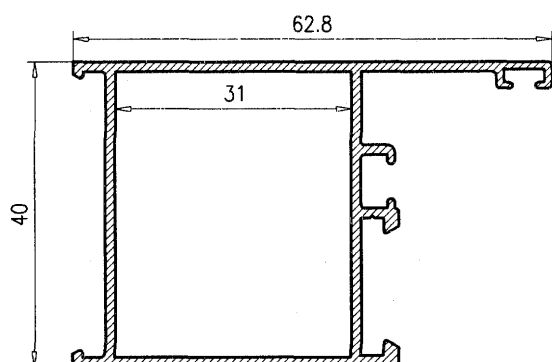
Marco Puerta 129280
