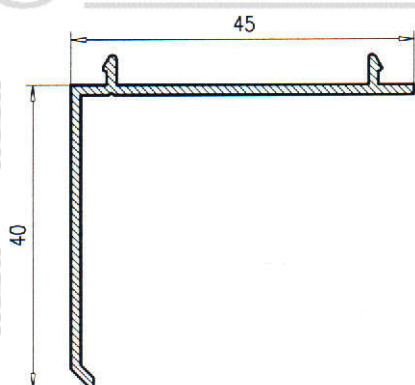
Premarco 40 040
