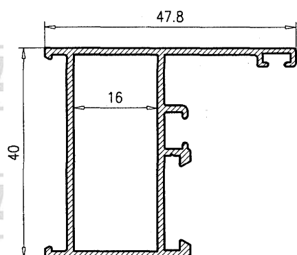
Marco Ventana 128280
