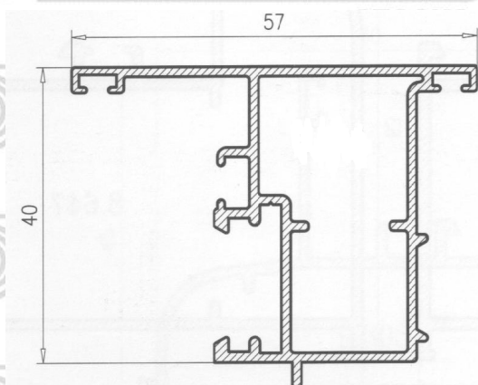
Marco Ventana 128280
