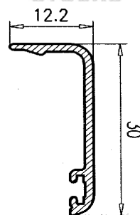
Premarco Cajón 30 039
