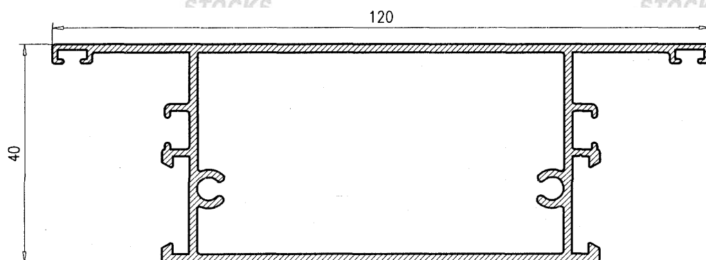
Pilastra Zócalo 129477
