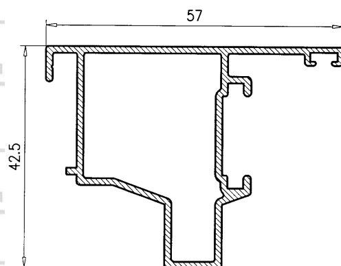
Perfil Pivote 128084
