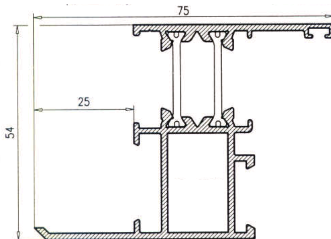
Marco Ventana c/premarco
