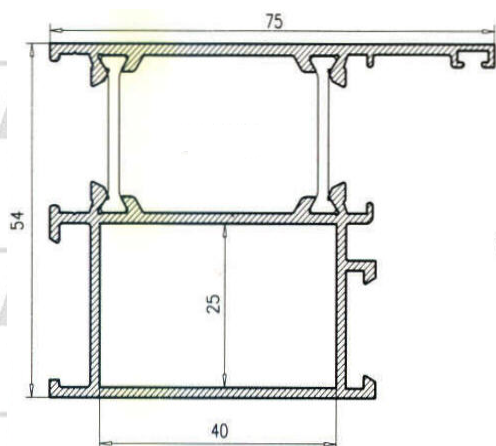
Marco Puerta
