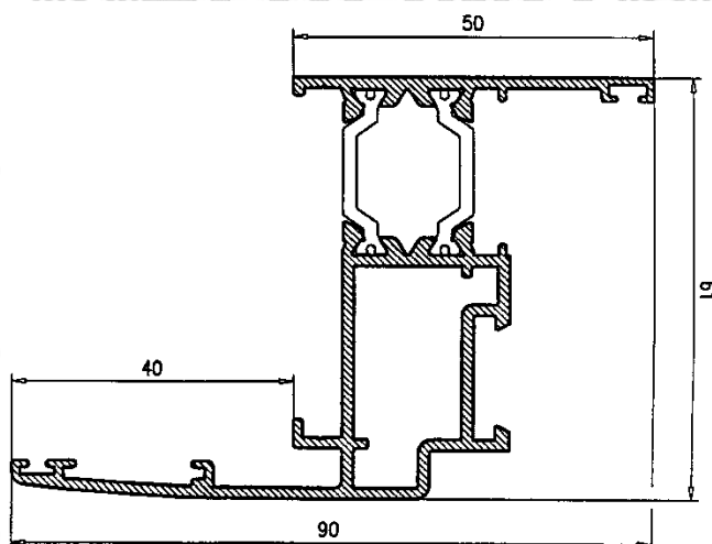
Marco Ventana con solape
