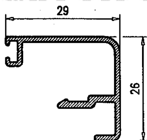
Junq. Base 29 hueco 21.5
