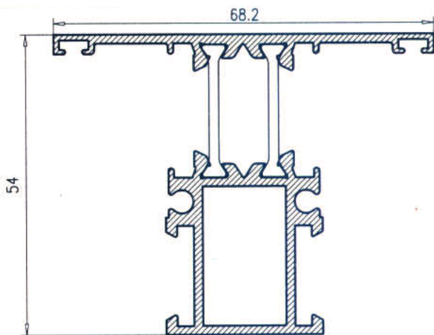
Pilastra Ventana
