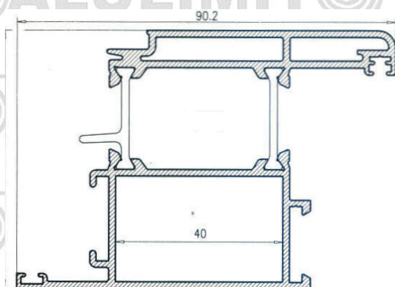
Hoja Puerta
