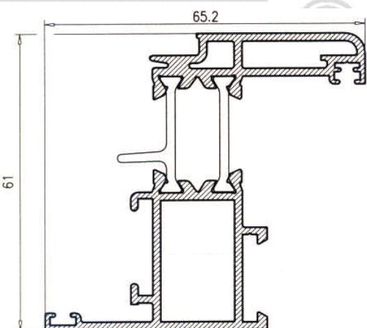
Marco Ventana
