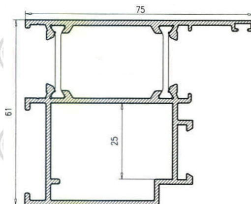
Marco Puerta Enrasado
