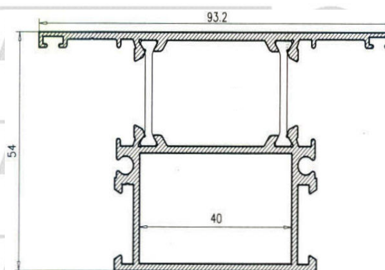
Pilastra Puerta
