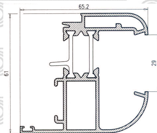
Hoja Ventana s/junquillo
