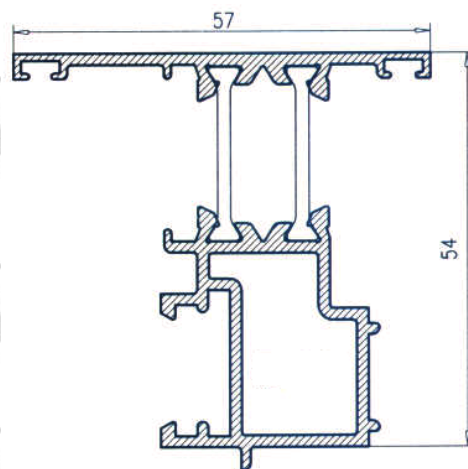
Esquinero 45
