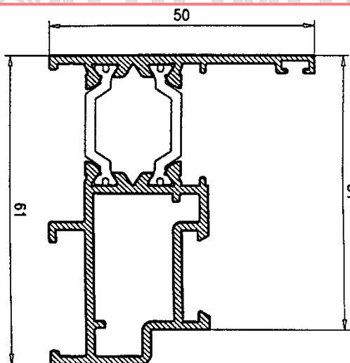
Marco Ventana
