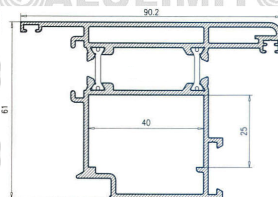
Hoja Apertura Exterior Puerta
