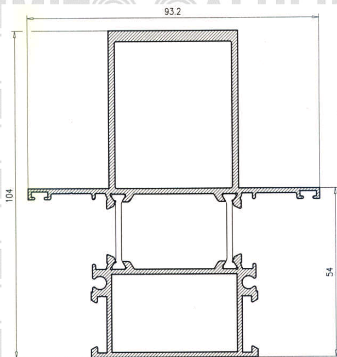
Pilastra Muro Cortina
