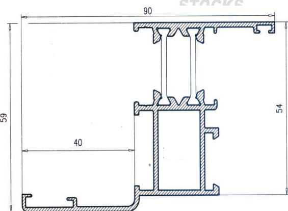
Marco Ventana Solape
