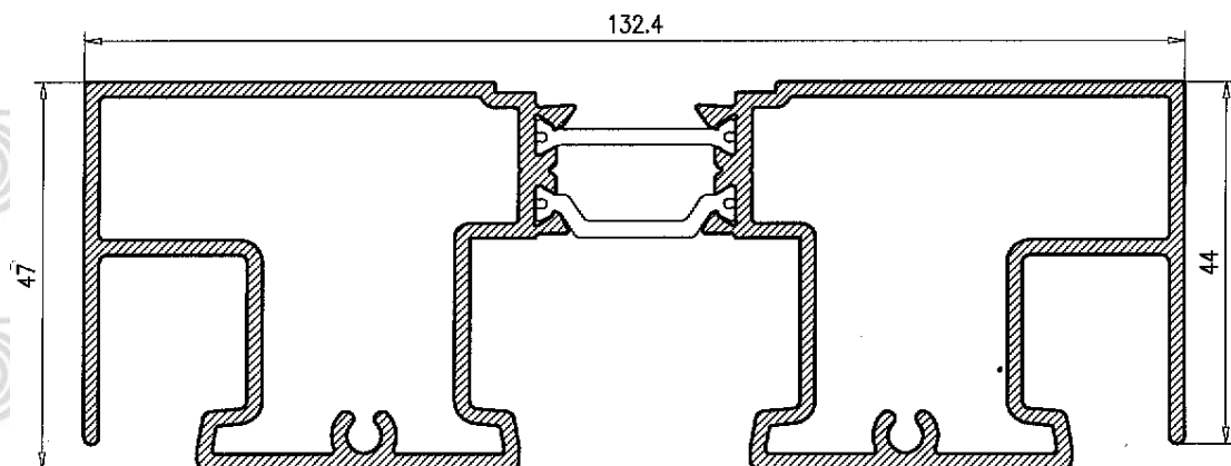
Marco Superior 60
