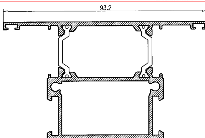
Pilastra Puerta 37580
