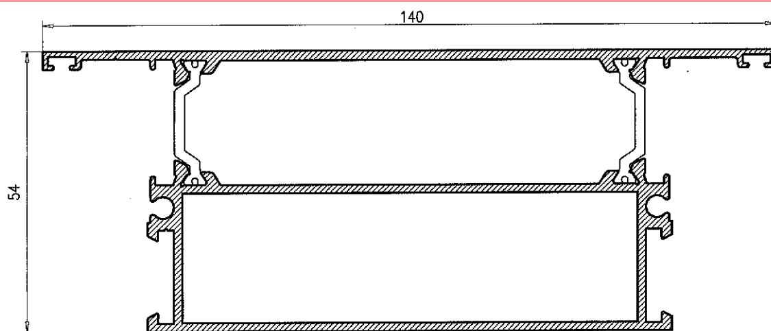
Pilastra Zócalo 37476
