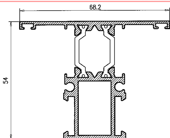
Pilastra Ventana 36580
