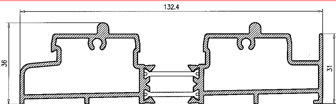
Marco Inferior 61
