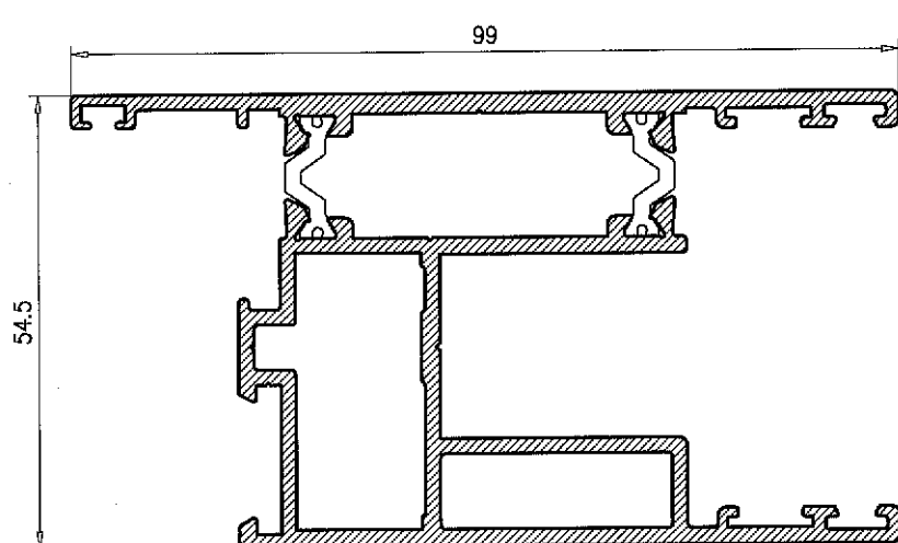
Hoja Perimetral 63
