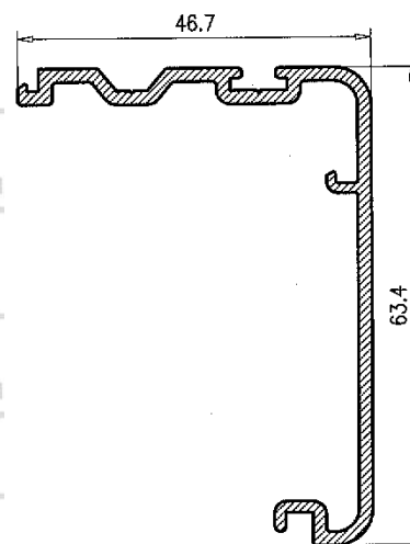
Cruce Central 66
