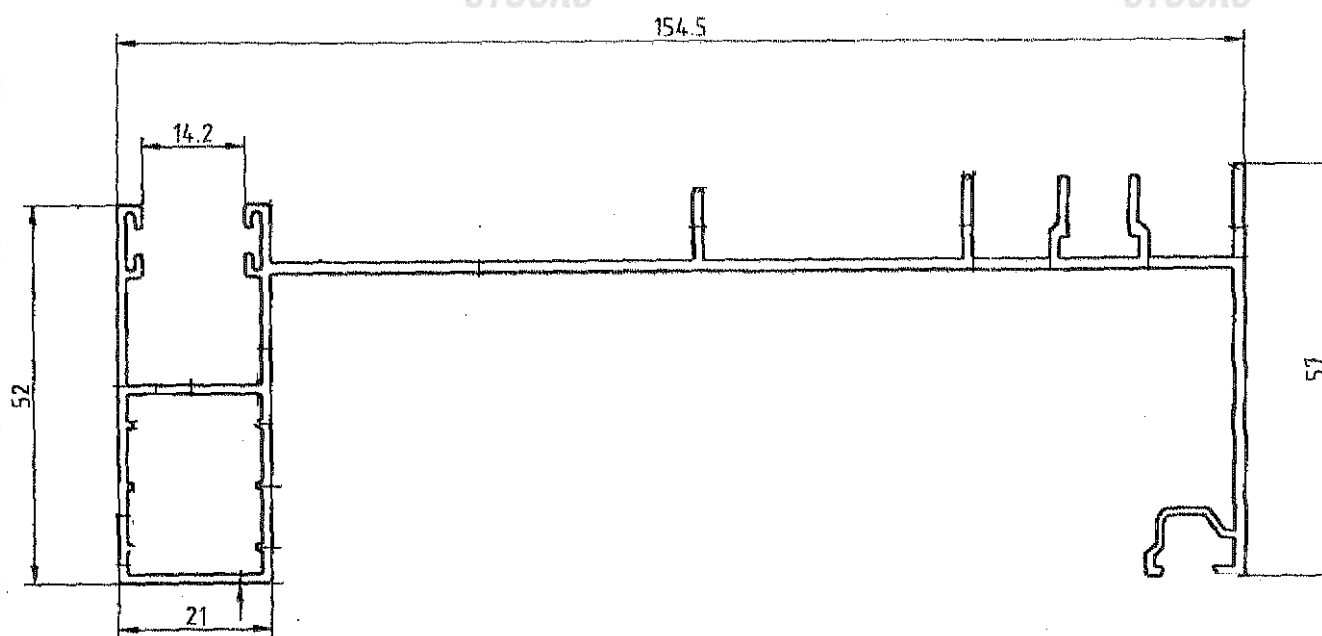
Marco Lateral Compacto Derecho 154.5 7206
