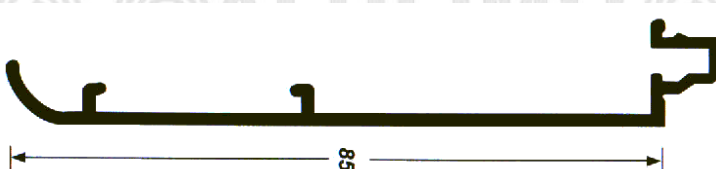
Premarco 85 7285
