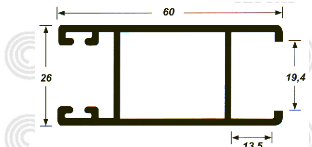
Hoja Lateral Climalit
