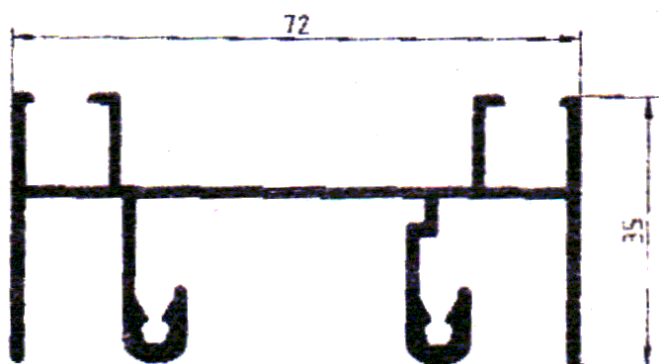
Marco Superior
