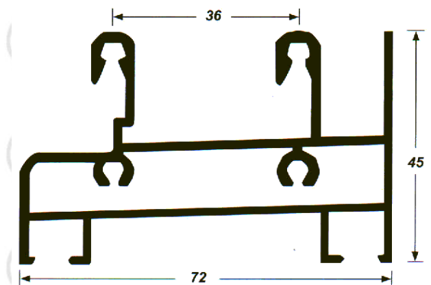
Marco Inferior
