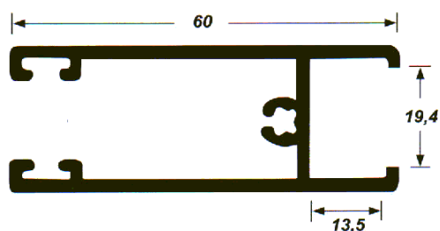
Hoja Rueda Climalit 7210
