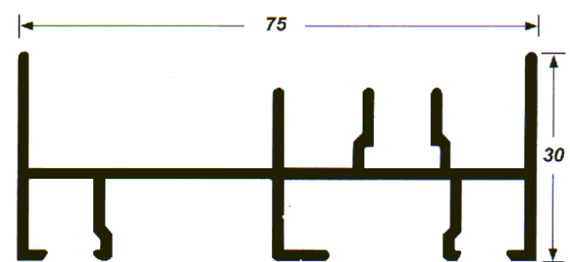
Marco Lateral Reforzado
