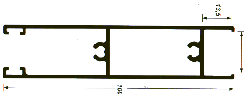
Zócalo Climalit 7220
