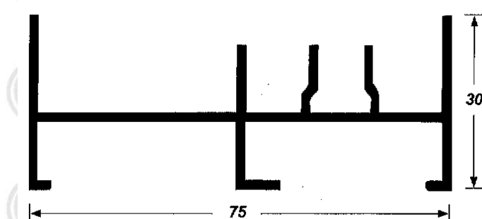
Marco Lateral Nuevo
