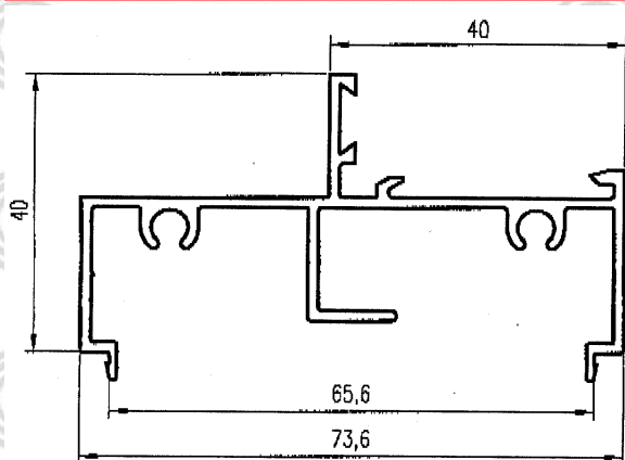
Marco Inferior c/refuerzo 812
