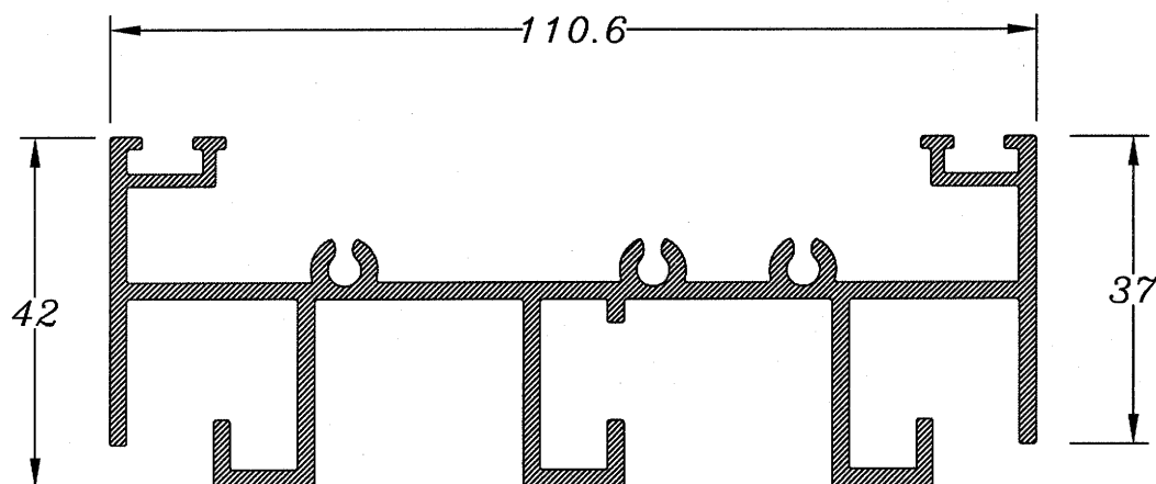
Marco Superior 3 carriles 821
