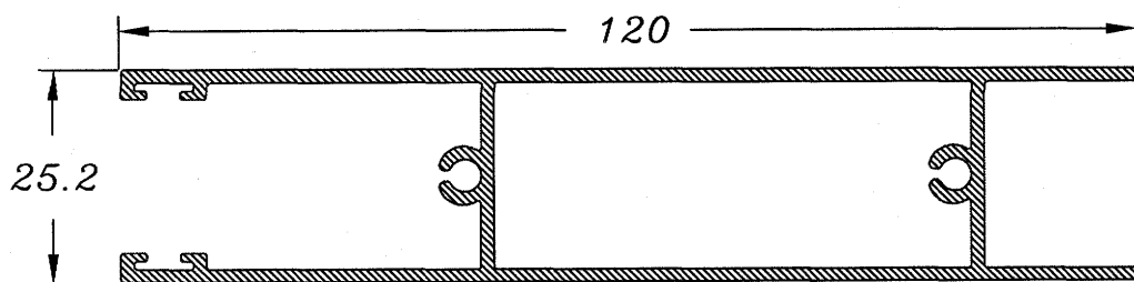
Zocalo Climalit 847
