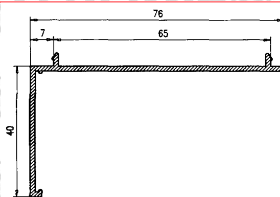
Premarco 40 045
