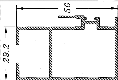
Hoja Lateral Normal 804
