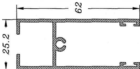
Hoja Central Normal 805
