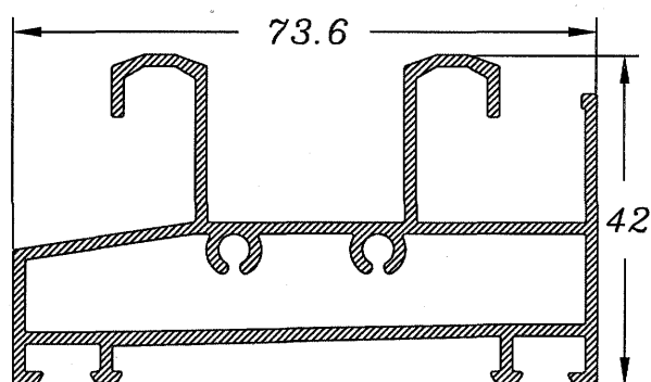
Marco Lateral c/pestaña 803
