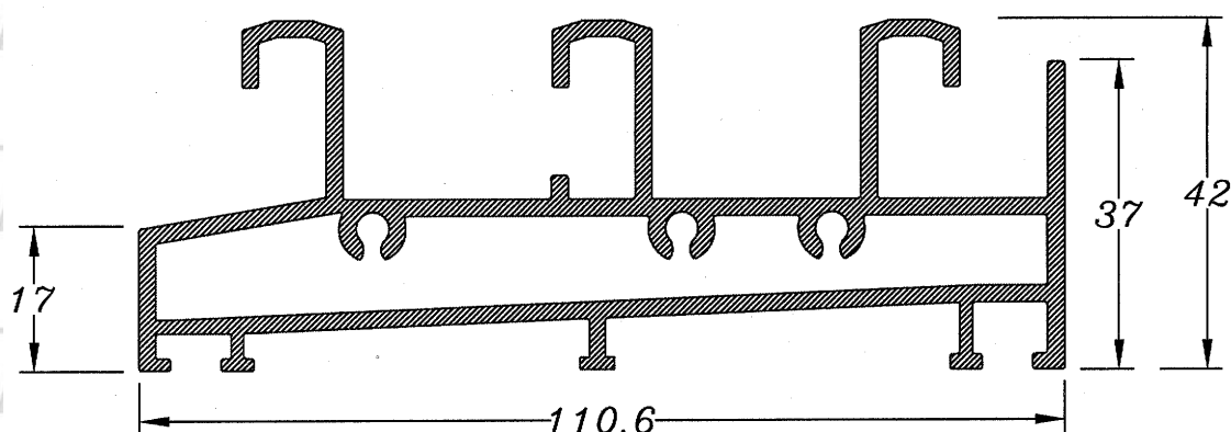
Marco Inferior 3 carriles 822
