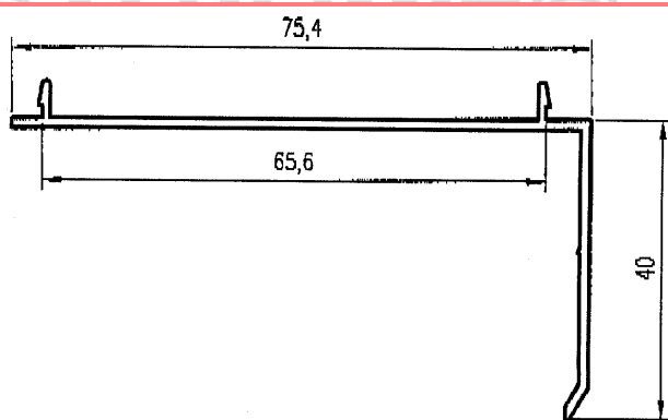
Premarco 40 biselado 046
