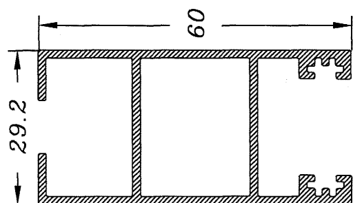
Hoja Lateral Normal 804
