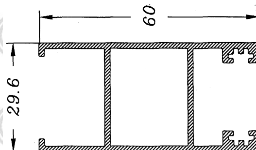
Hoja Lateral Climalit 834
