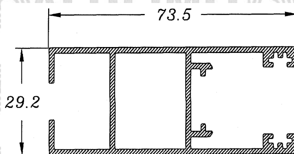
Marco Superior c/refuerzo 811
