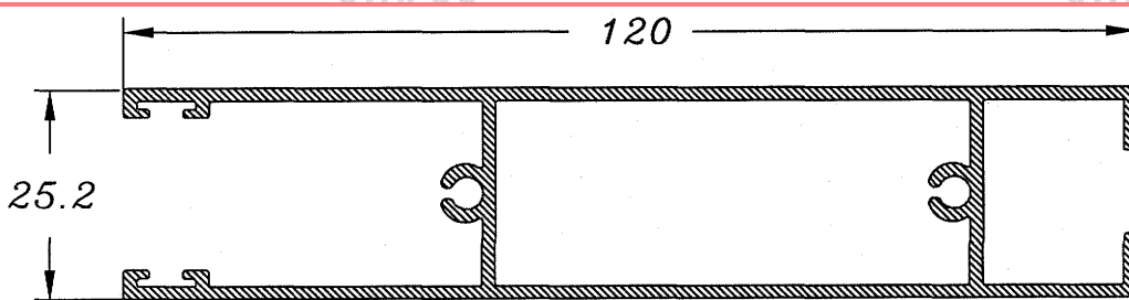
Zocalo Normal 846
