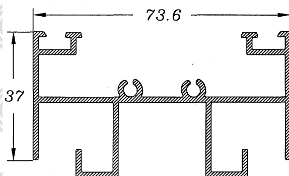
Marco Superior c/refuerzo 811
