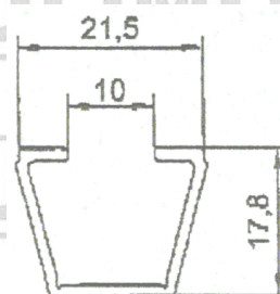
U Compensadora 815
