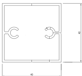
Cuadrado 40 aut.
