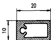
R 20*10 aut.
