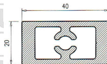
R. 40*20 aut.
