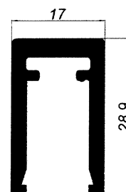
U para acristalar
