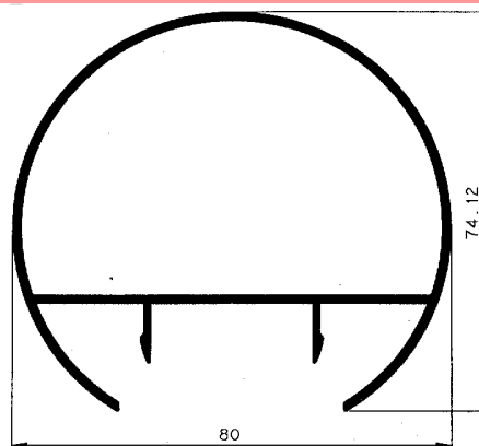
Pasamano Redondo 80
