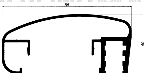
Pasamano 86 europeo acristalar
