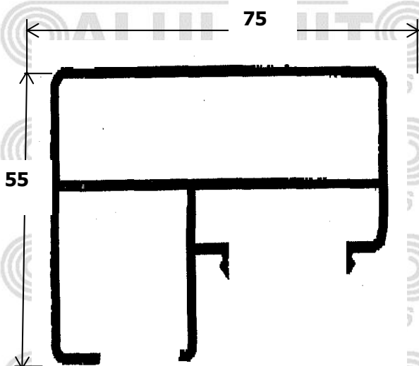
Pasamano Cristal
