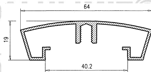
Pasamano autorroscado
