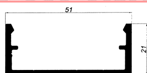
U Pasamano de 51
