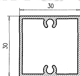
Cuadrado 30 aut.
