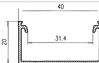
Forma U 20
