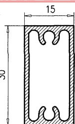
R 30*15 aut.
