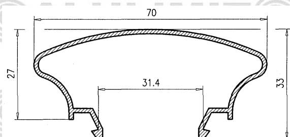
Pasamano Barandilla
