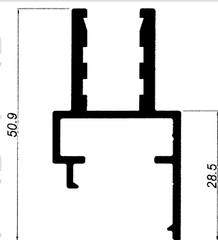
Anclaje Cristal
