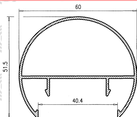
Pasamano Redondo 60
