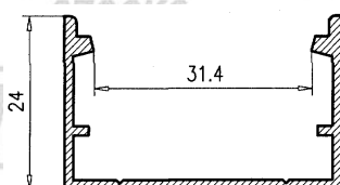
Forma U 25
