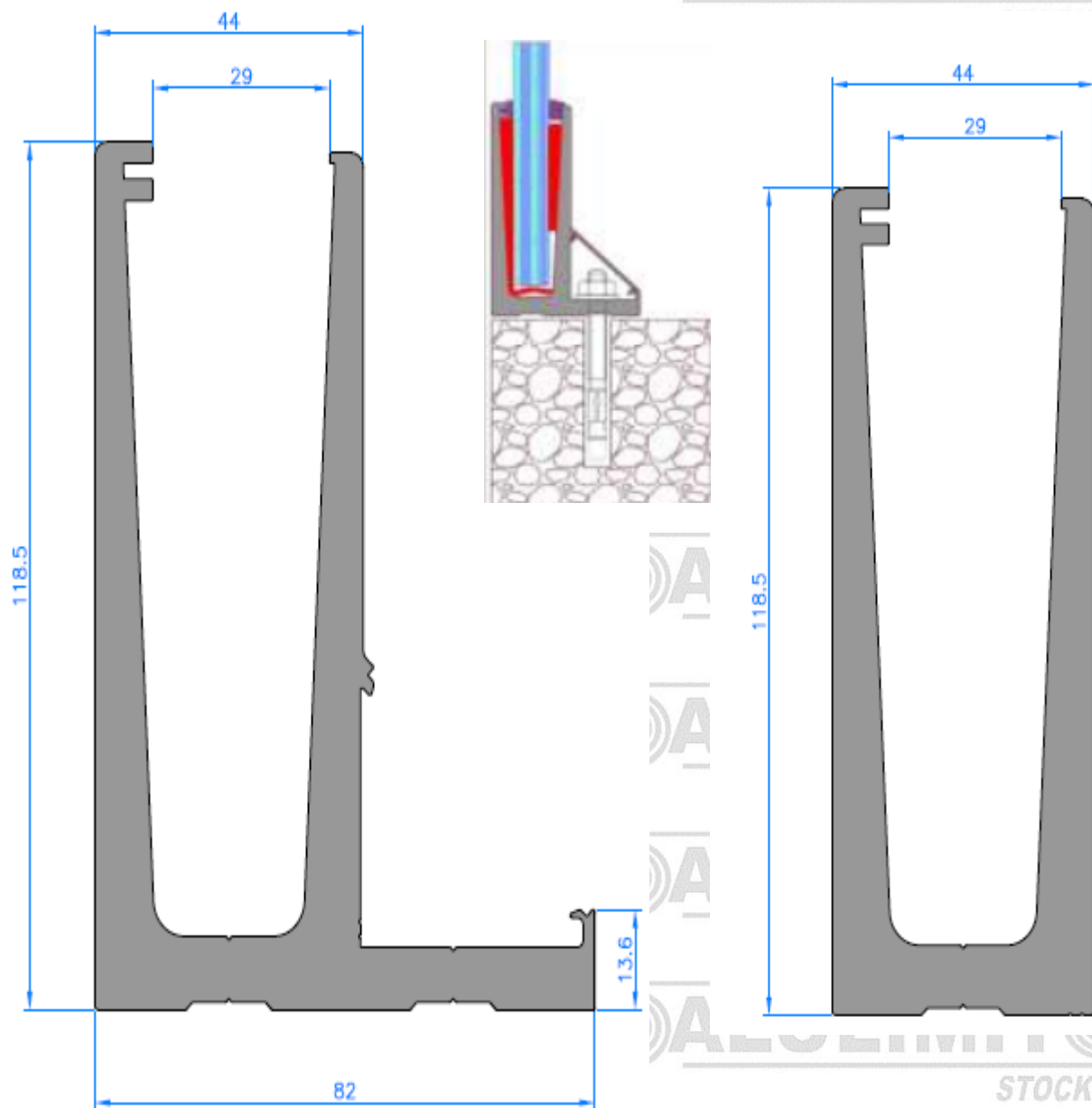
Perfil sujeción al suelo 816
