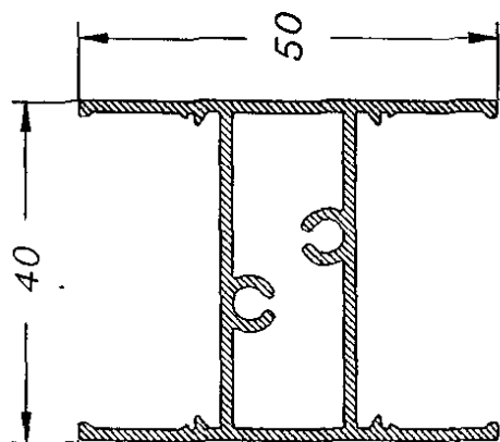
Parteluces
