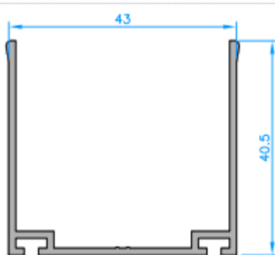
U Compensadora 40
