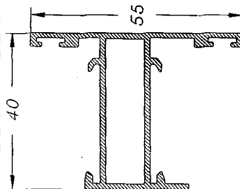
T inversora
