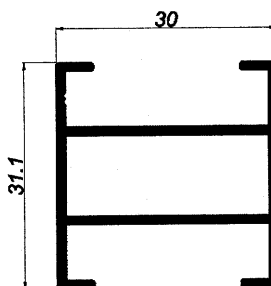
Pilastra de 30
