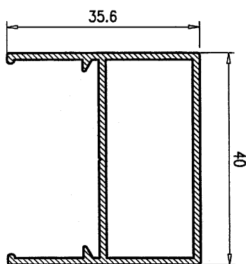
Marco Celosía 24
