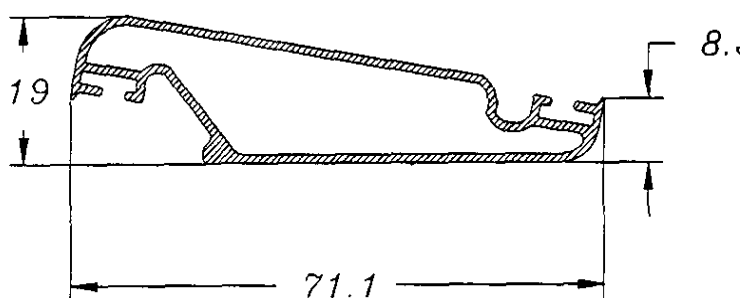
Lama Perla 70
