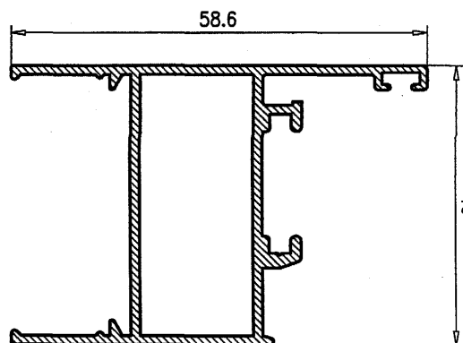
Hoja europeo 25
