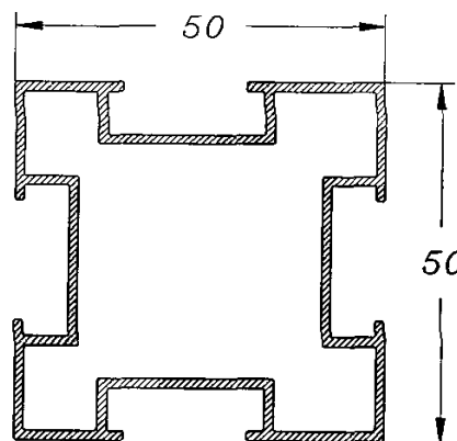
Perfil 4 Salidas 502
