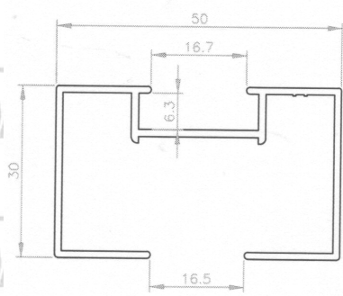
Perfil 1 Salida 03112
