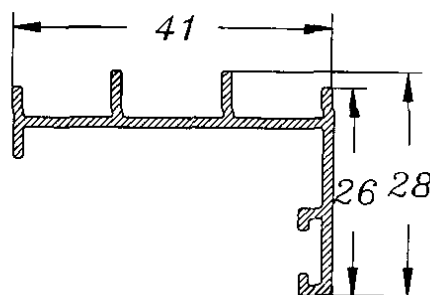
Perfil Cerco 504
