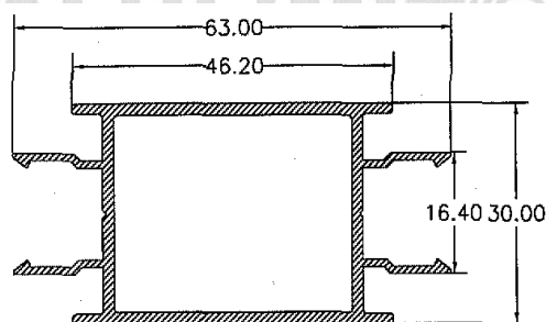
Mampara doble 508
