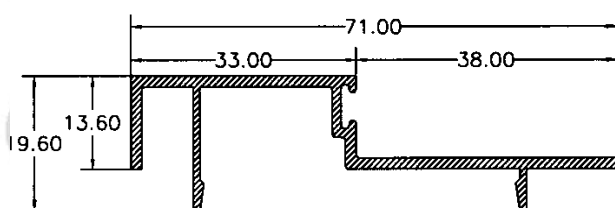
Acople puerta 510
