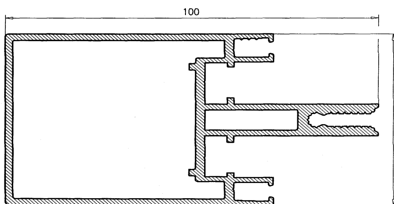
Travesaño 73 606
