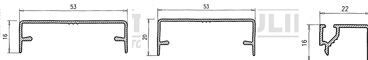
Tapeta Travesaño 16 600 Tapeta Montante 20 601 Junquillo 16 604
