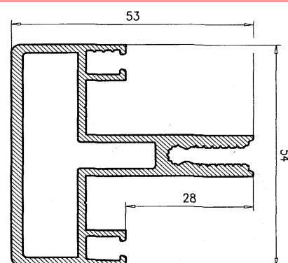
Base Acristalamiento 603
