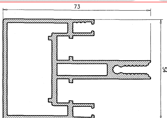
Tapeta Montante 46 602
