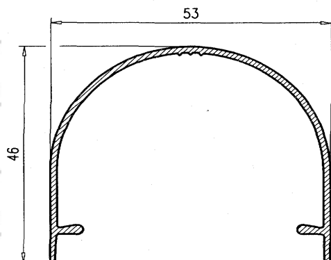
Tapeta Montante 46 602
