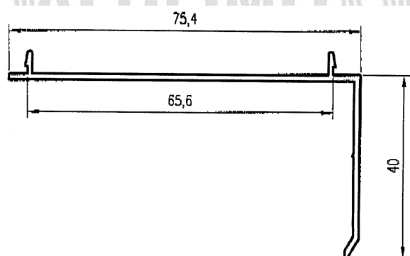
Premarco 40 biselado 046
