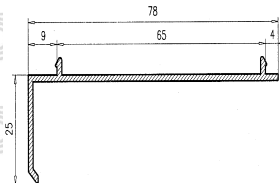
Premarco de 25 922
