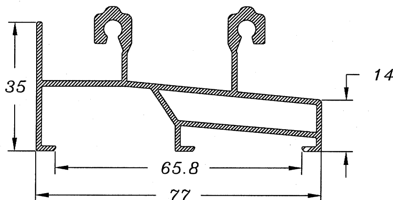
Marco Inferior 91
