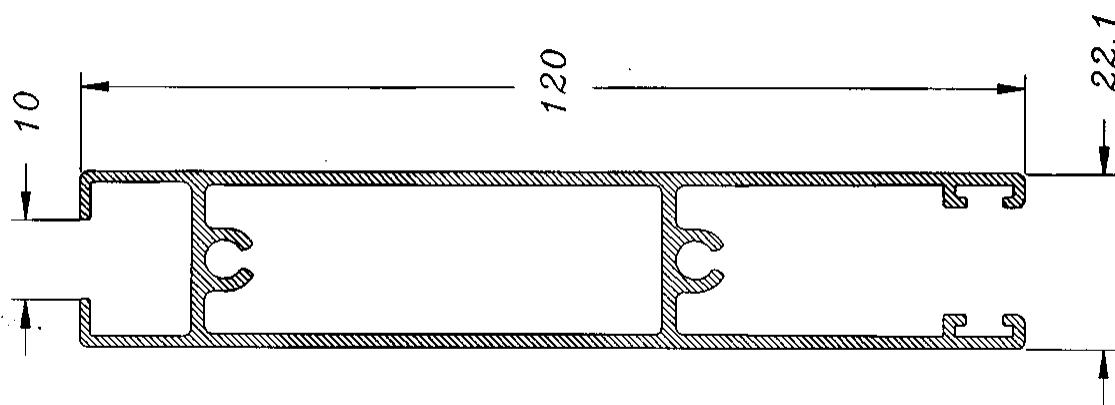
Zócalo Normal 97
