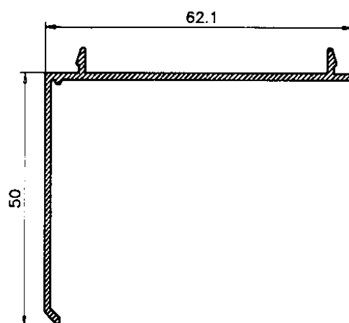
Premarco 50 044
