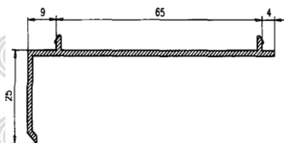
Premarco 25
