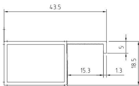
Premarco obra 36. PLADUR 43.5 514
