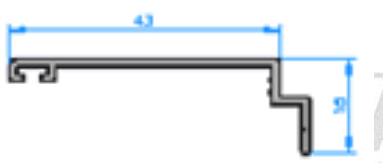
Premarco 43 atornillado
