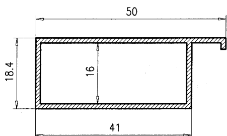
Premarco obra 50 507
