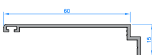
Premarco 60 atornillado
