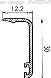
Tapa Cajón 039
