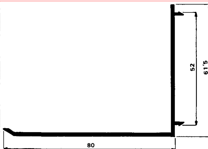
Premarco 40 040
