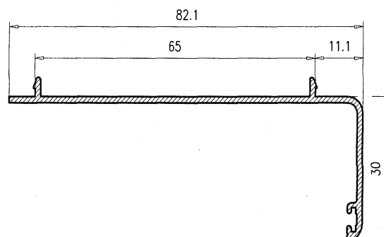
Premarco 30 042
