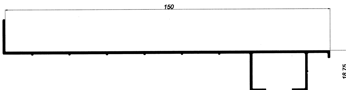
Premarco obra de 150 511
