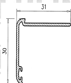
Premarco 30 041
