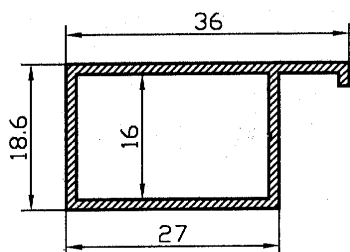
Premarco obra 36 506
