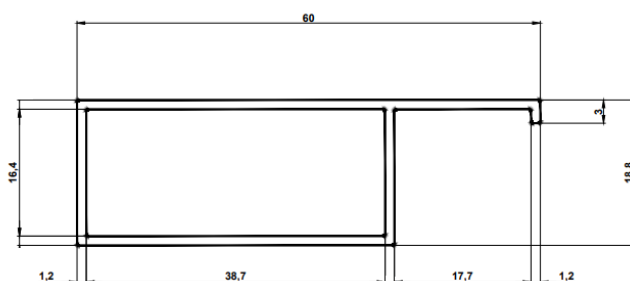
Premarco obra 50. PLADUR 60 515
