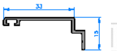
Premarco 33 atornillado
