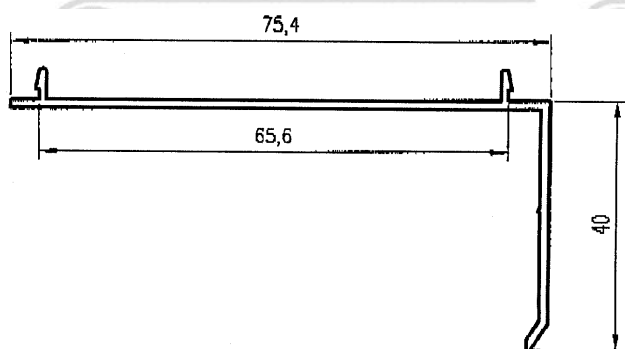
Premarco 80 atornillado
