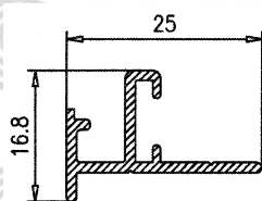
Solape 40 031
