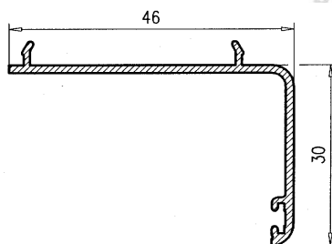
Premarco 30 041
