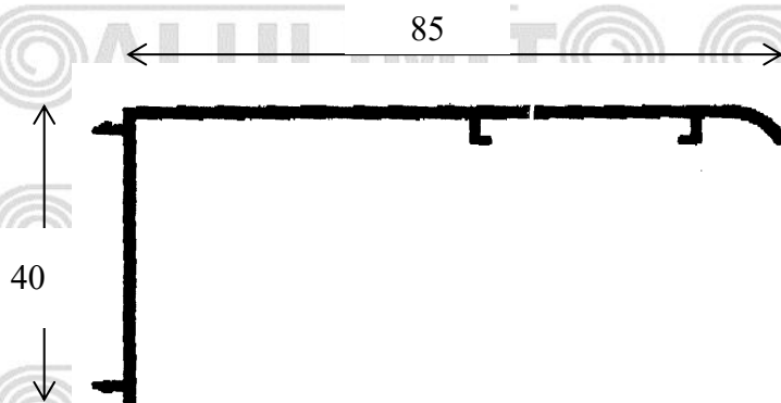
Premarco 40 biselado
