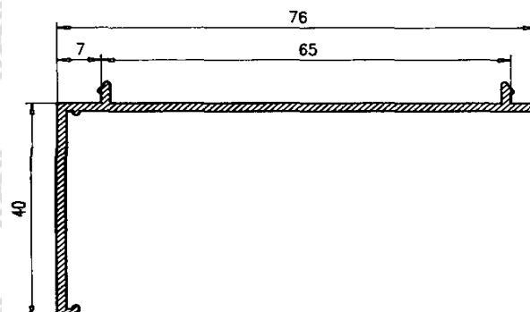
Premarco 25
