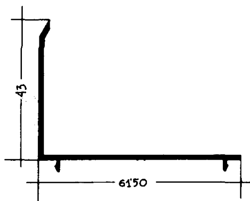
Premarco 43 043
