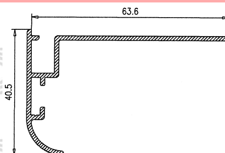
Solape 40 Cataluña 032
