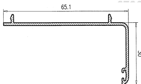
Premarco 30 042
