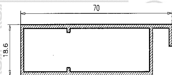
Premarco obra 50 507
