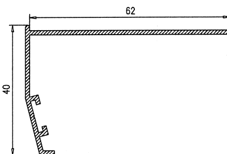
Solape 40 recto 033
