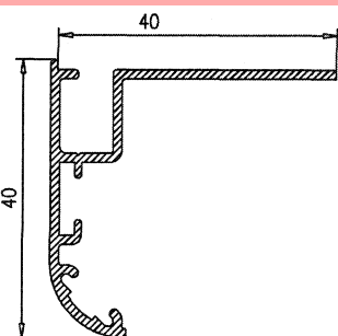
Solape 40 031
